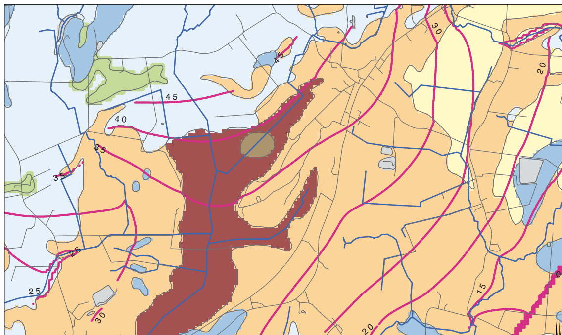
Figur 1. Grundvattennivåer (rosa ekvipotentiallinjer) vid befintligt uttag. Naturlig grundvattenbildning. Skala ca 1:20 000.
