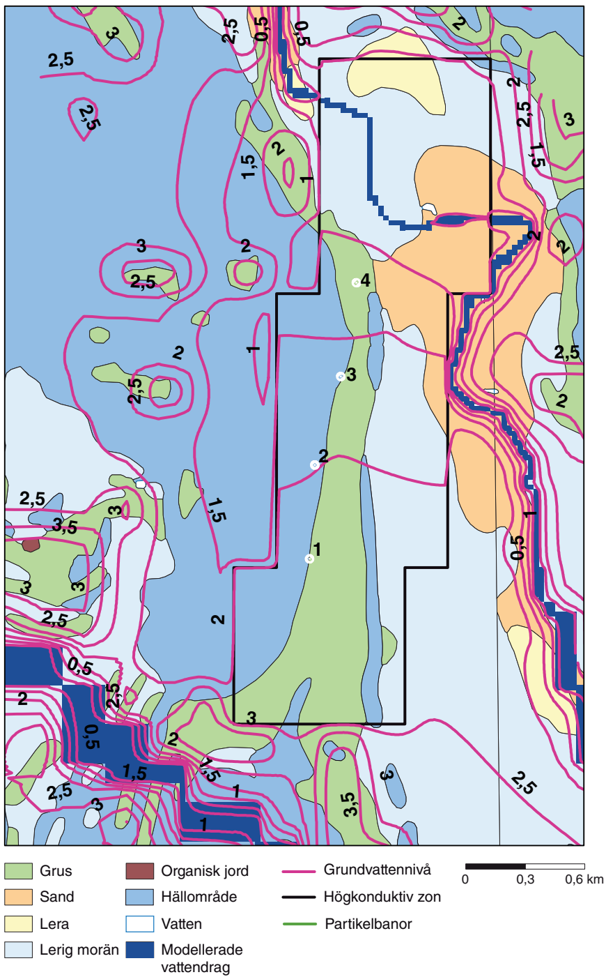
Figur 4. Grundvattenavsänkning jämfört med dagens situation efter 10 års drift av ett scenario med halvårsvis förstärkt infiltration (vinter) i utspridda dammar och halvårsvis ökat uttag (sommar). Grundvattenavsänkningen (lila ekvipotentiallinjer) påverkar ett större område runt infiltrationsbassängerna och brunnarna.
