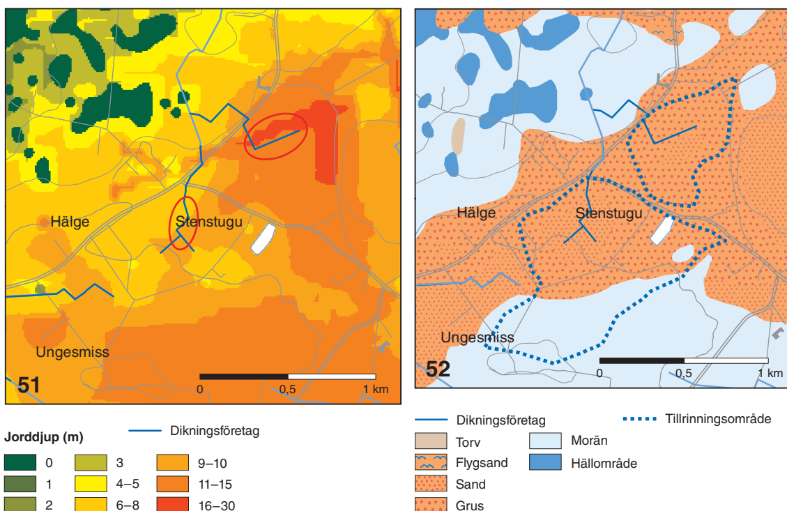
Figur 51. Jorddjupskarta över vattentäkstens närområde. Röda ovaler symboliserar möjligt område för potentiell våtmarksanläggning.
