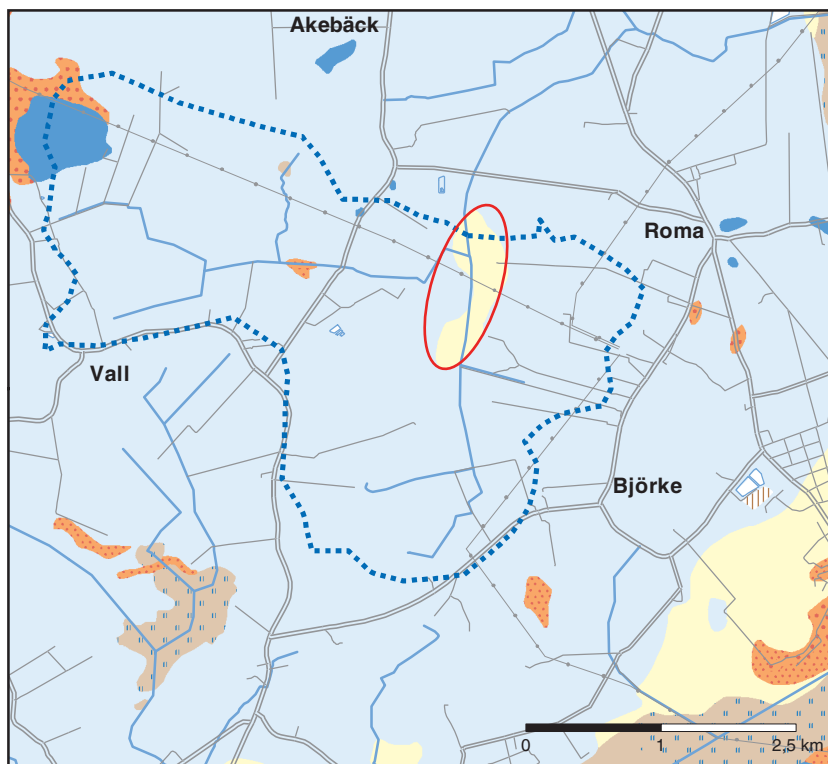
Figur 49. Figuren visar vattentäktbrunnarna vid Roma. Uppskattat tillrinningsområde för det dike som rinner strax väster om Busarvebrunnarna, samt möjligt område för potentiell våtmarksanläggning (röd oval). Underlaget är SGUs jordartskarta.
