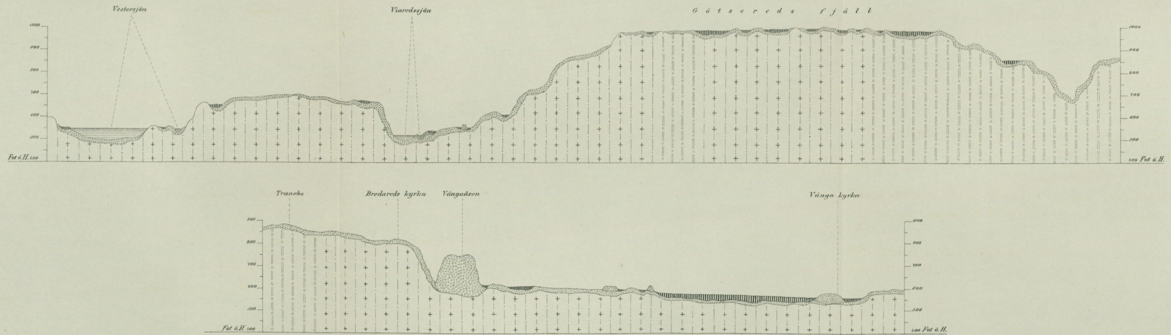
Profil N o 2 öfver Viaredsjön, Götsereds fjäll, Bredareds och Vänga kyrkor.
