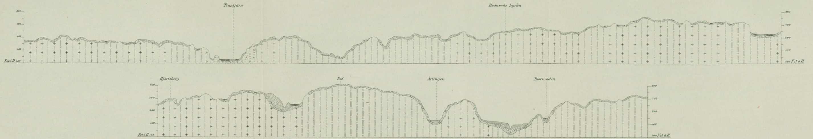
Profil N o 1 öfver Trantjärn, Hedareds kyrka och Ärtingen.
