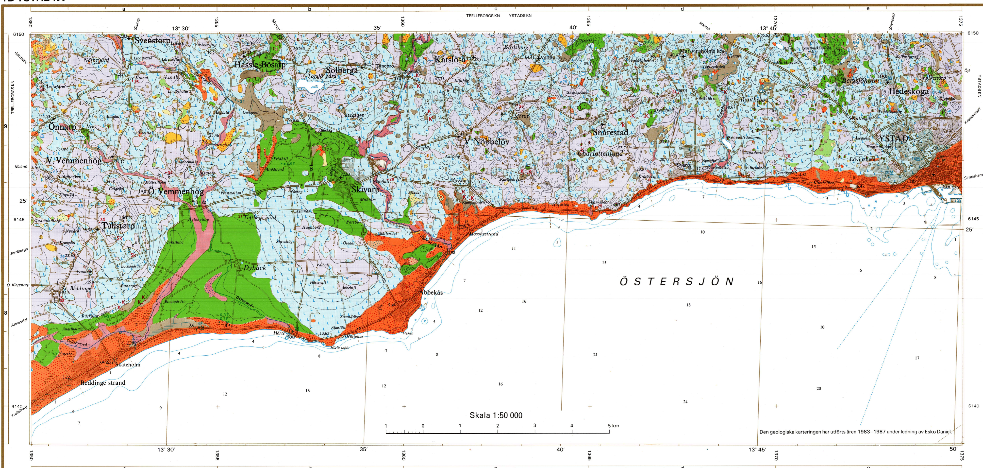
BERGGRUNDSKARTA PRE-QUATERNARY ROCKS
