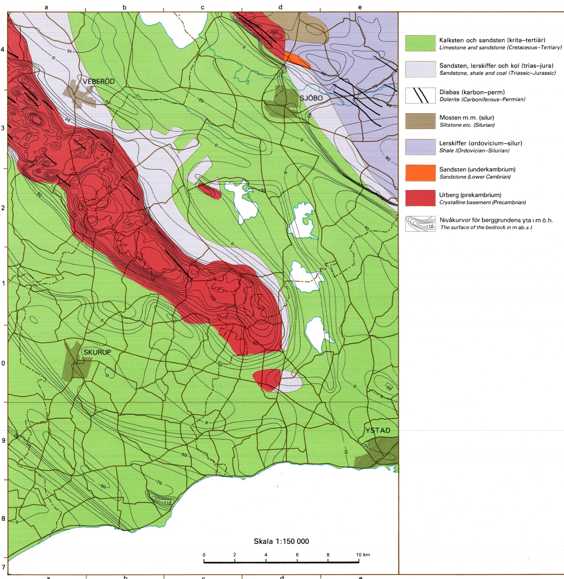
BERGGRUNDSKARTA PRE-QUATERNARY ROCKS
