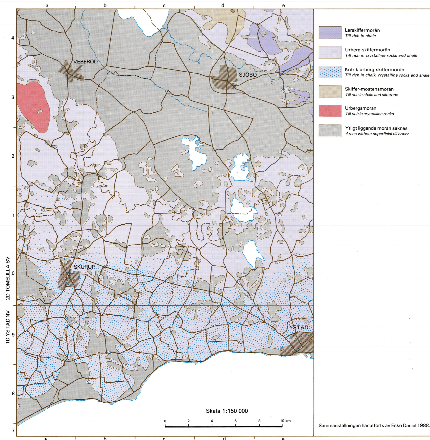
UTBREDNINGEN AV OLIKA MORÄNTYPER EFTER LITOLOGISK SAMMANSÄTTNING DISTRIBUTION OF TILLS WITH DIFFERENT LITHOLOGICAL COMPOSITION
