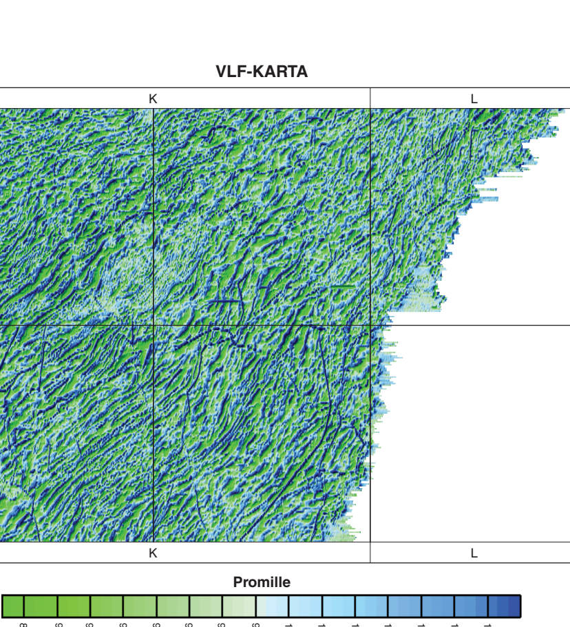
VLF-karta över kartbladsområdet 21K Roberfors och 21L Ånåset (skala 1:600 000). Kartan visar den relativa totalintensiteten av det sekundärt inducerade elektromagnetiska fältet...
