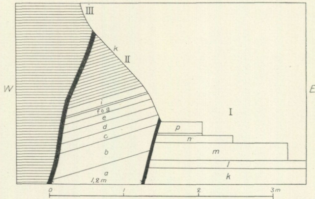
Textfig. 3. Section from the western part of the locality E 21 a, Fågelsång.
