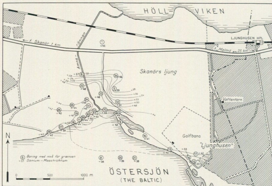
Fig. 5. Kotekort over Skanörhalvöen med boringerne og grænsen Danium-Maastrichtium. Map of the Eastern Skanör peninsula with the wells and the contour of the boundary Danian-Maastrichtian.
