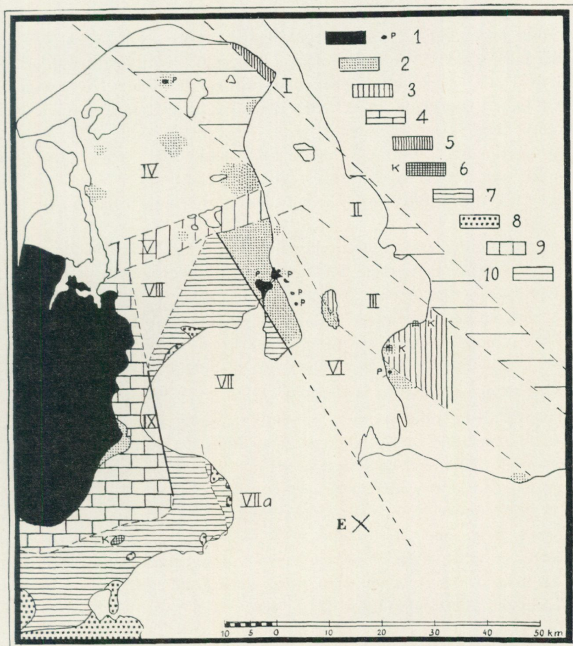
Fig. 1. Undergrundskort over det østlige Sjælland med tilgrænsende Omraader. Romertallene I-IX angiver i Teksten omtalte Omraader. 1. Paleocænforekomster. 2. Kalksandsomraader. 3, 4 og 5. Bryozokalk, for 3 og 4 de yngre Lag. 6. Koralkalk. 7. Bryozokalk (ældre Lag). 8. Skrivekridt. 9. Søndersødalen. 10. Alnarpdalen. Den svært optrukne Linje mellem Omraaderne VI og VII og VII og IX angiver Brudlinjer. Rette, stiplede Linjer Brudlinjer af mere usikker Karakter. E. Epicentret for Jordskælvet d. 1. November 1930 (efter I. Lehmann (2)). Kortet udarbejdet med delvis Benyttelse af de af V. Milthers (1908 og 1935) og J. P. J. Ravn (1922) udgivne Kort. Efter Rosenkrantz 1938.
