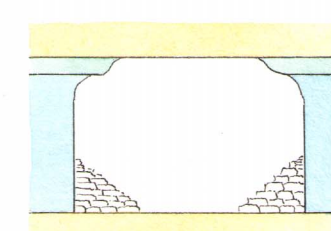
Trärprofil af holort i nedre flöts. Trärprofil af lerort i nedre flötsen.
