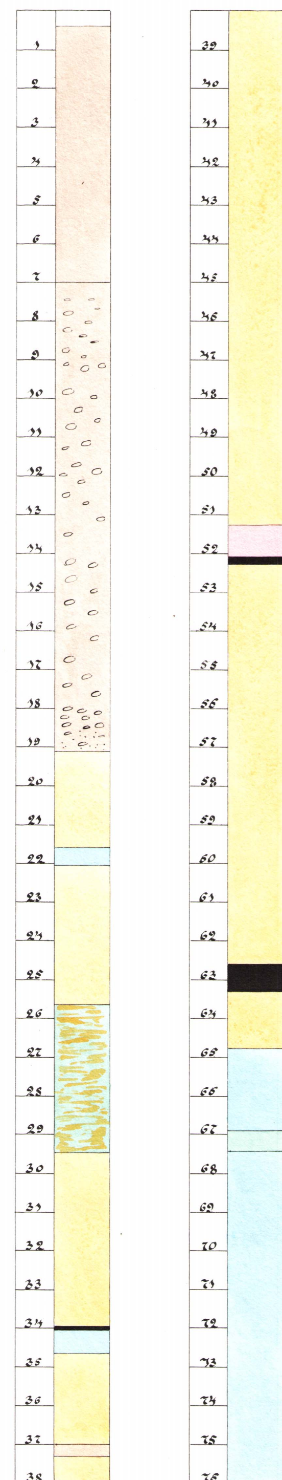
Profil genom Schakt N o 1. Skala 1:500
