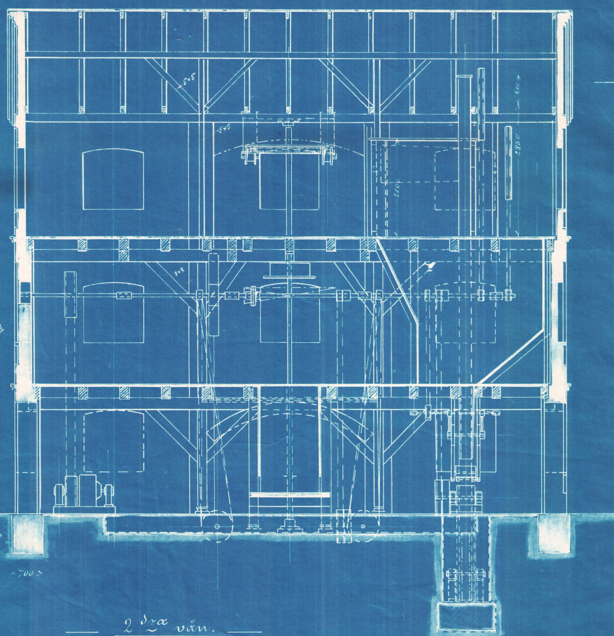
Snitt C-D
