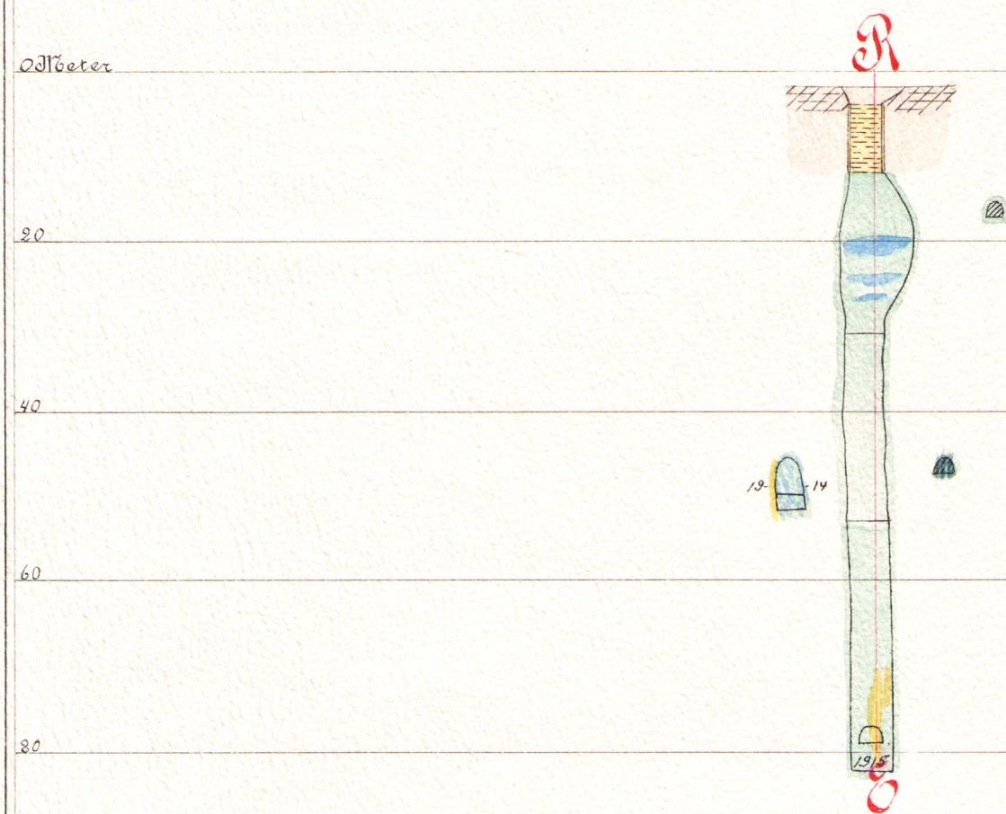
Längdprofil efter SS
