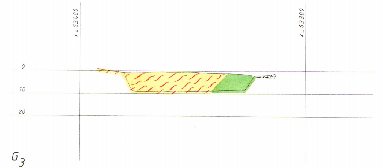
Vertikalskärning 93700 y
