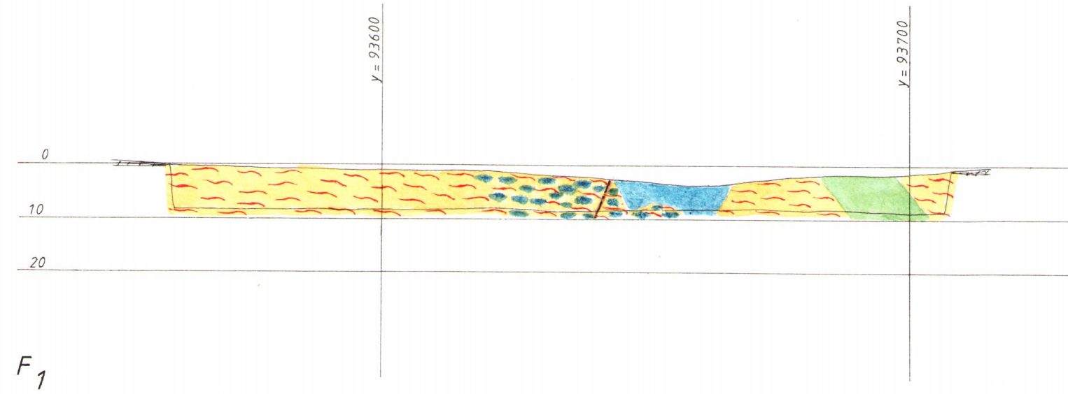
Längdprojektion A-B
