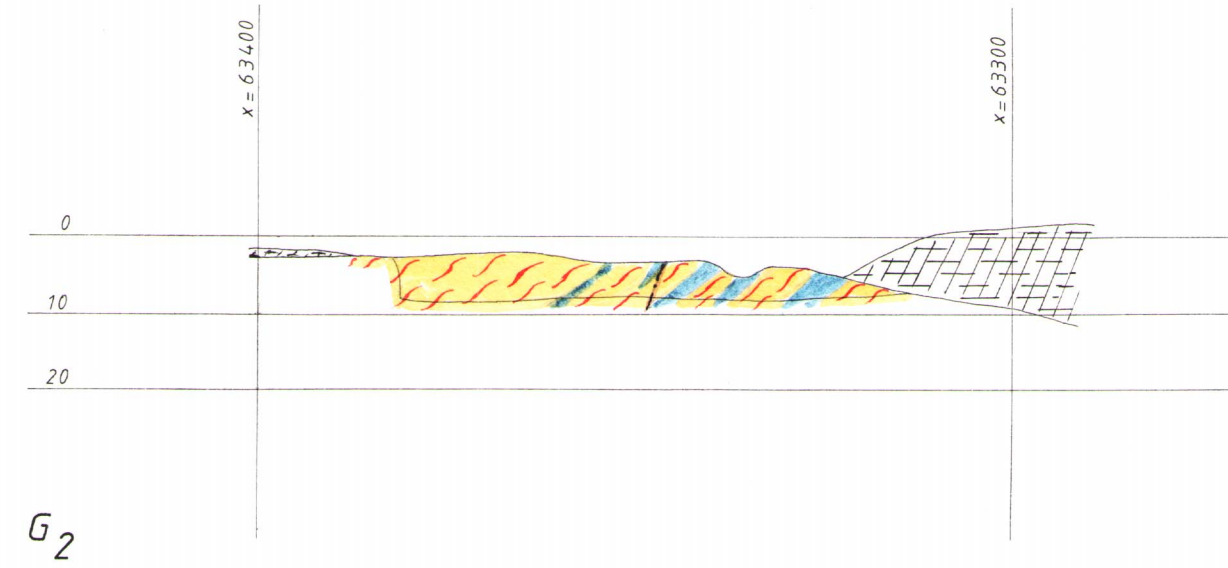
Vertikalskärning 93650 y
