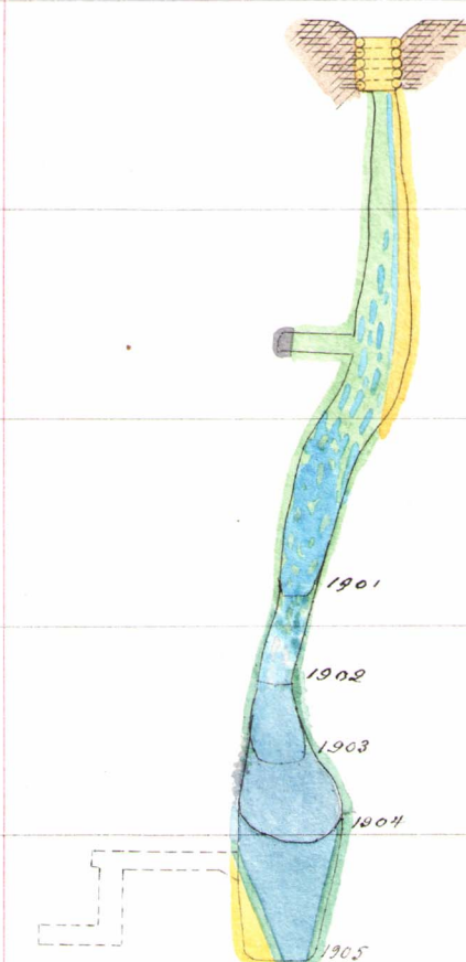
Trängprofil efter CD
