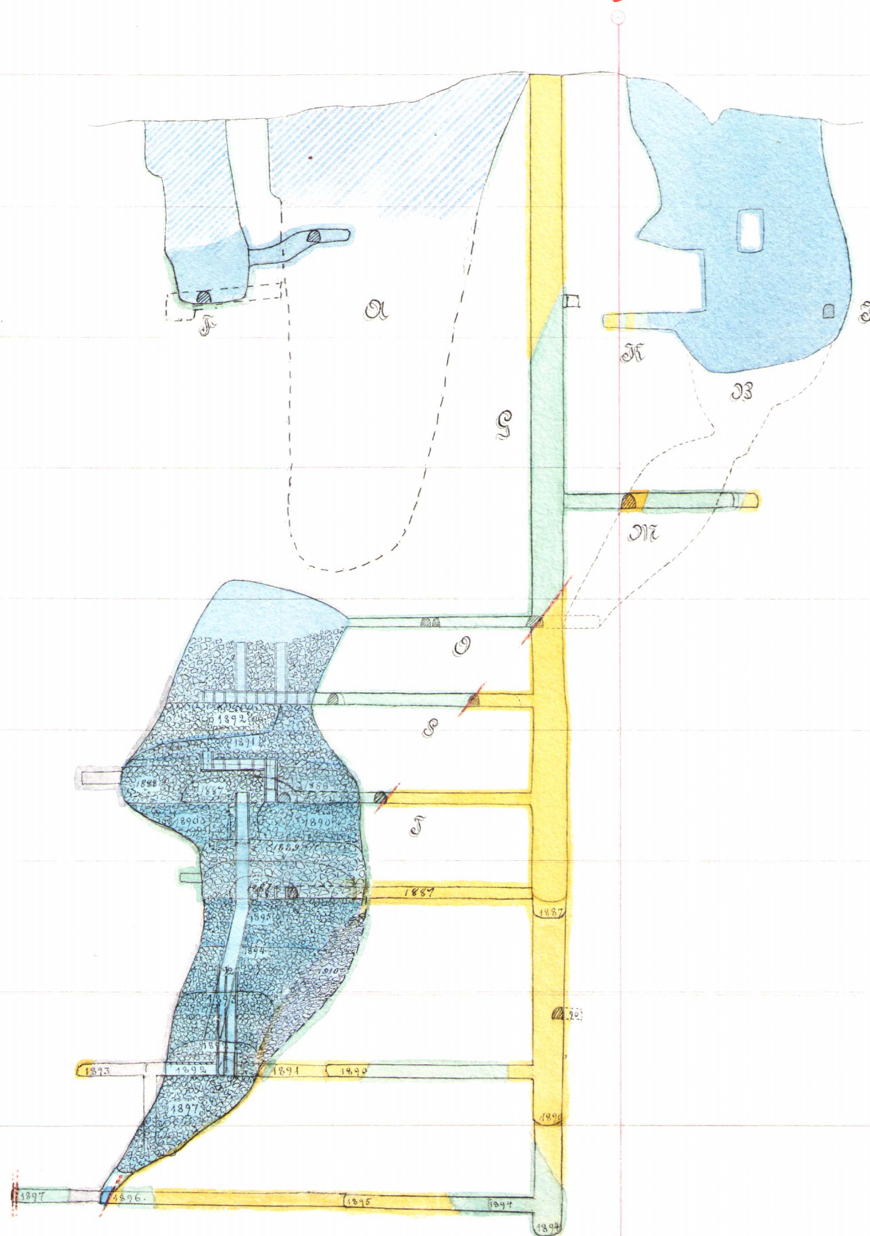
Projektioner af Grufvornas liggande vägg på vertikalplanet \alpha' \beta'
