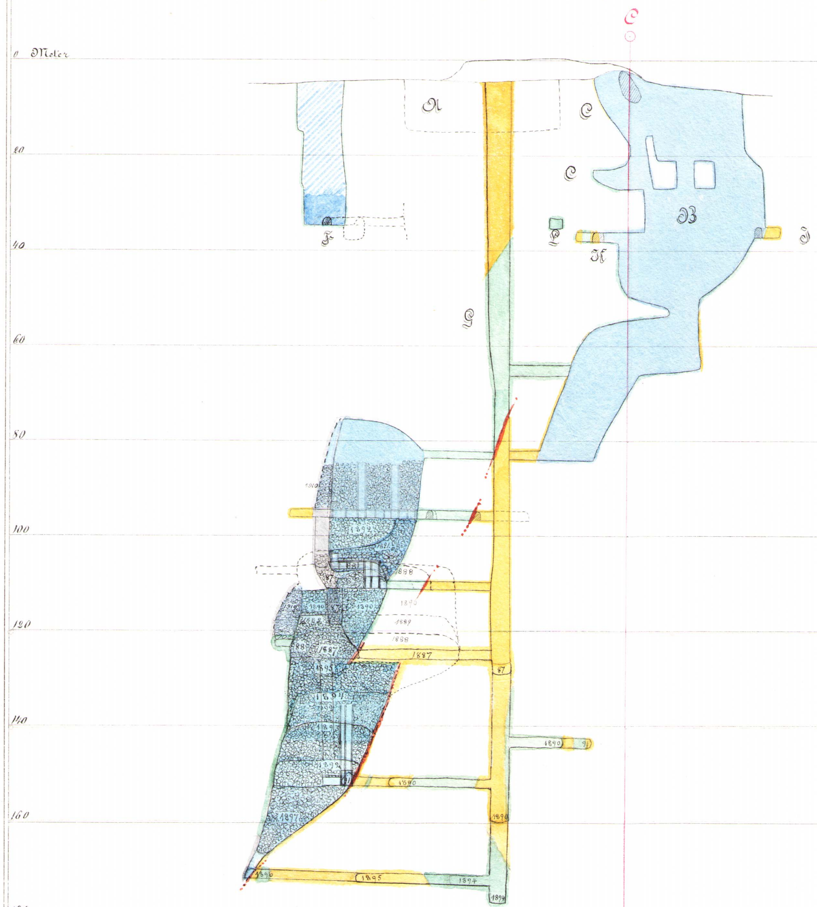
Projektion af Sikbergsgrufvans liggande vägg på vertikalplanet A B
