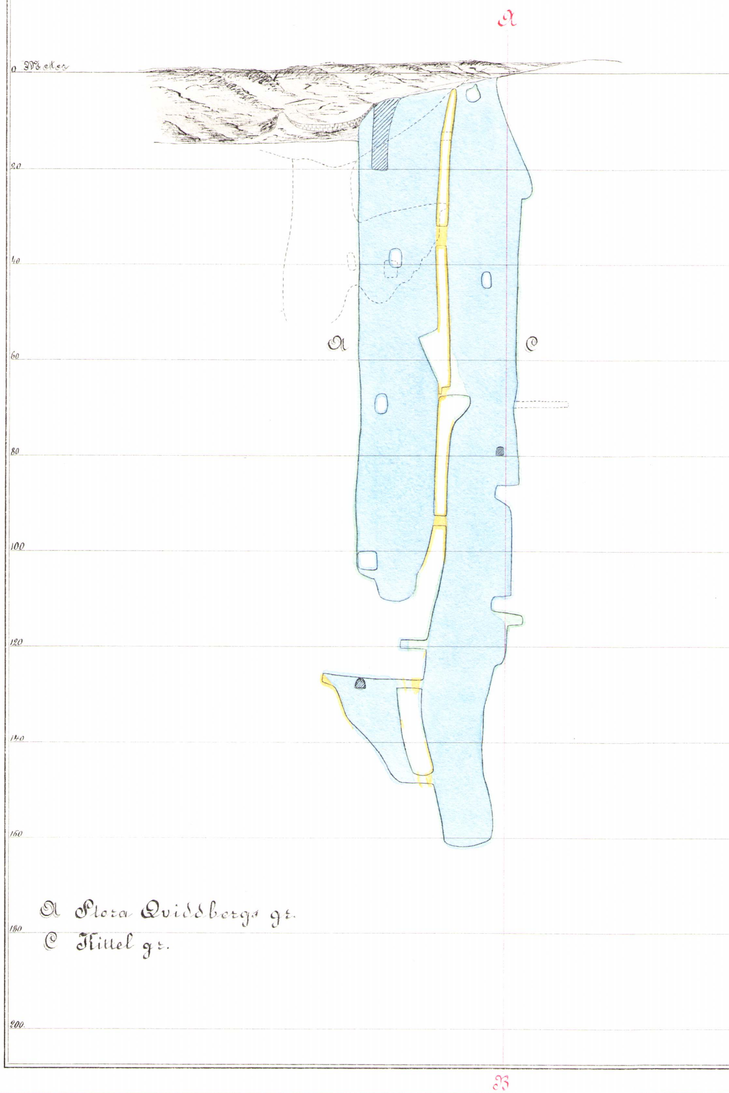
Projektion af Stora Qviddbergsgruvans liggande vägg på vertikalplanet D-C
