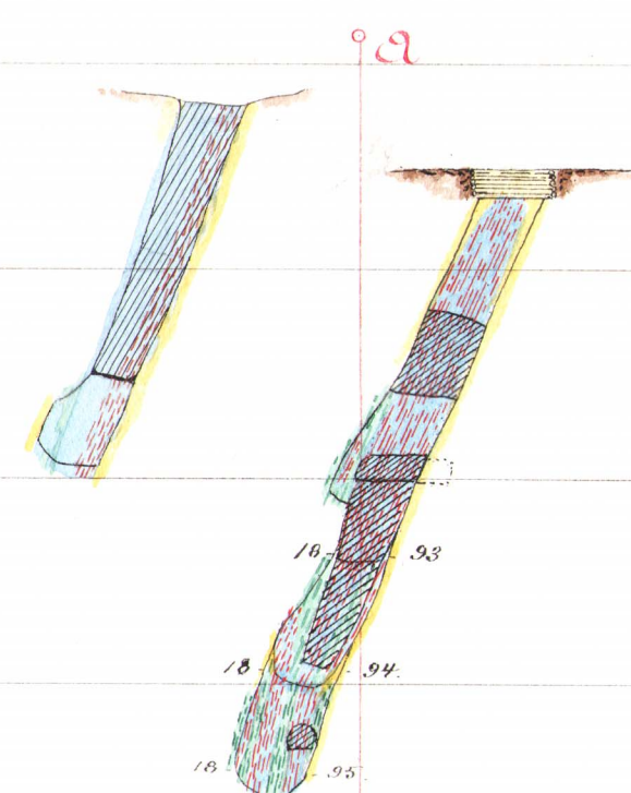
Snärprofil efter CD och EF
