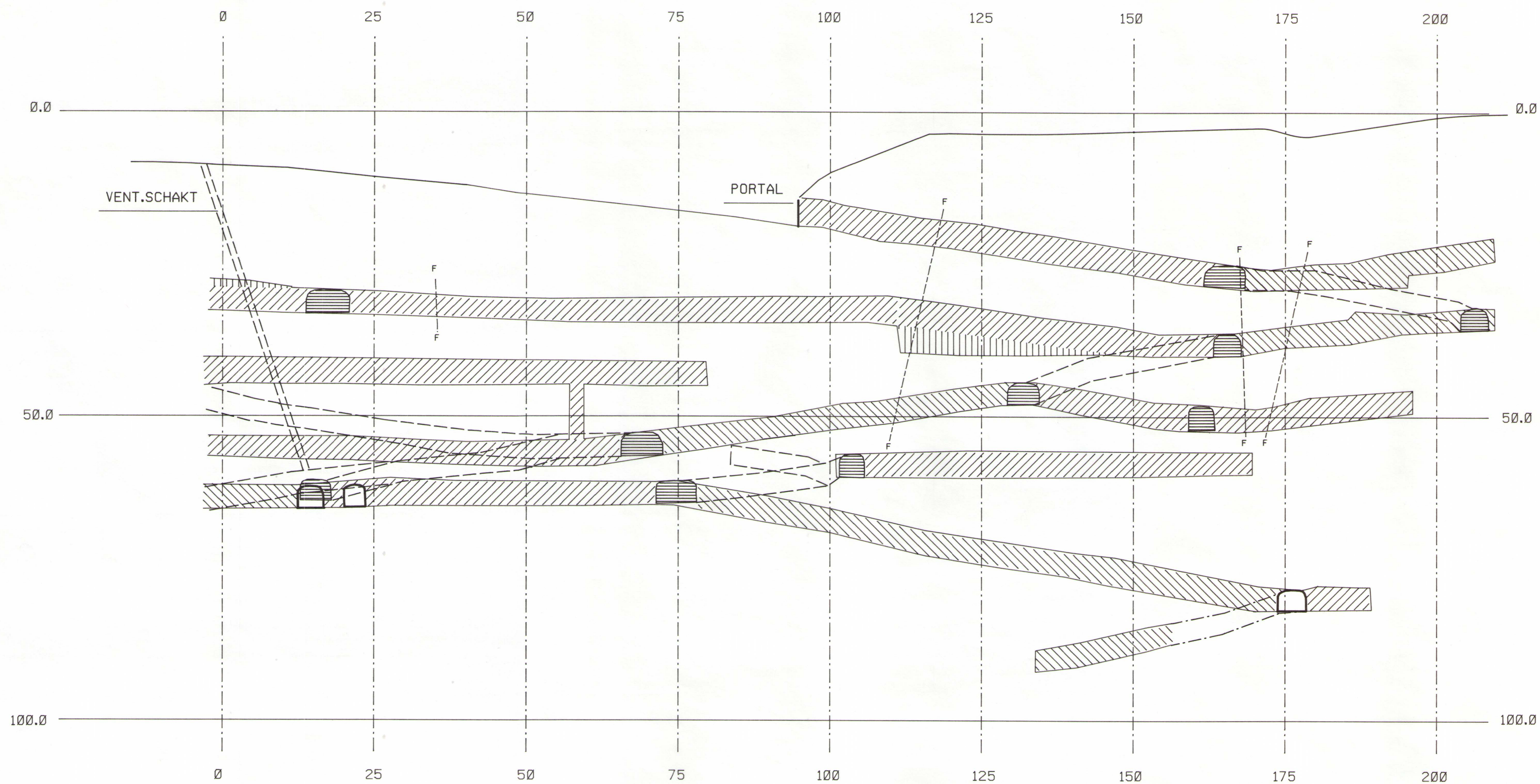
LOVISAGRUVAN LÄNGDPROJEKTION B - C Huvudmalmen Skala 1:500
