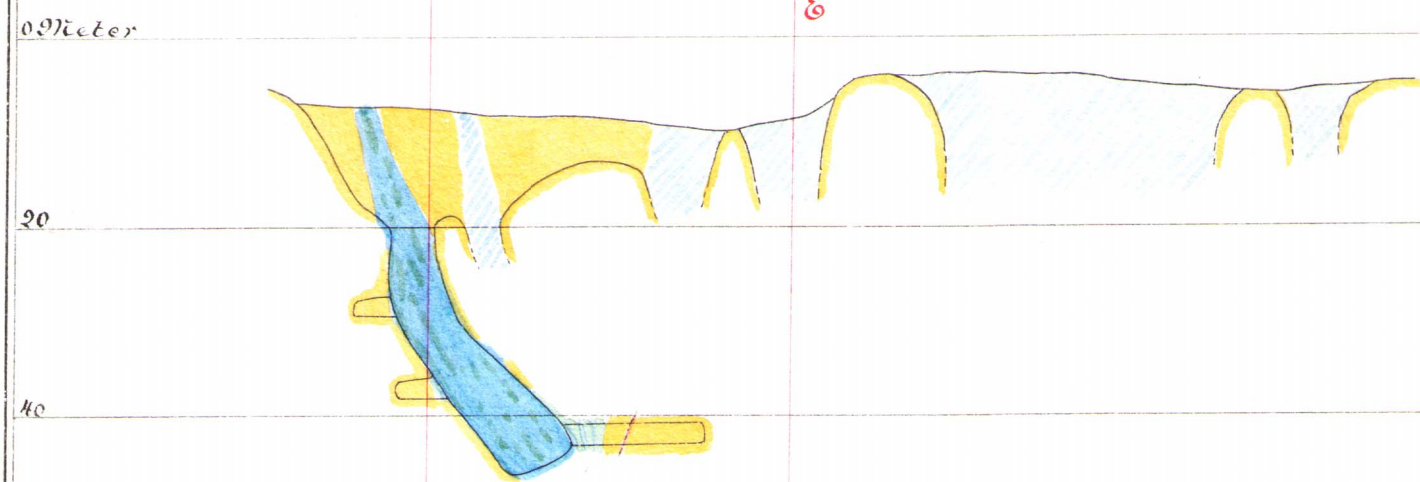
Längdprofil efter A B (Södra linserna)
