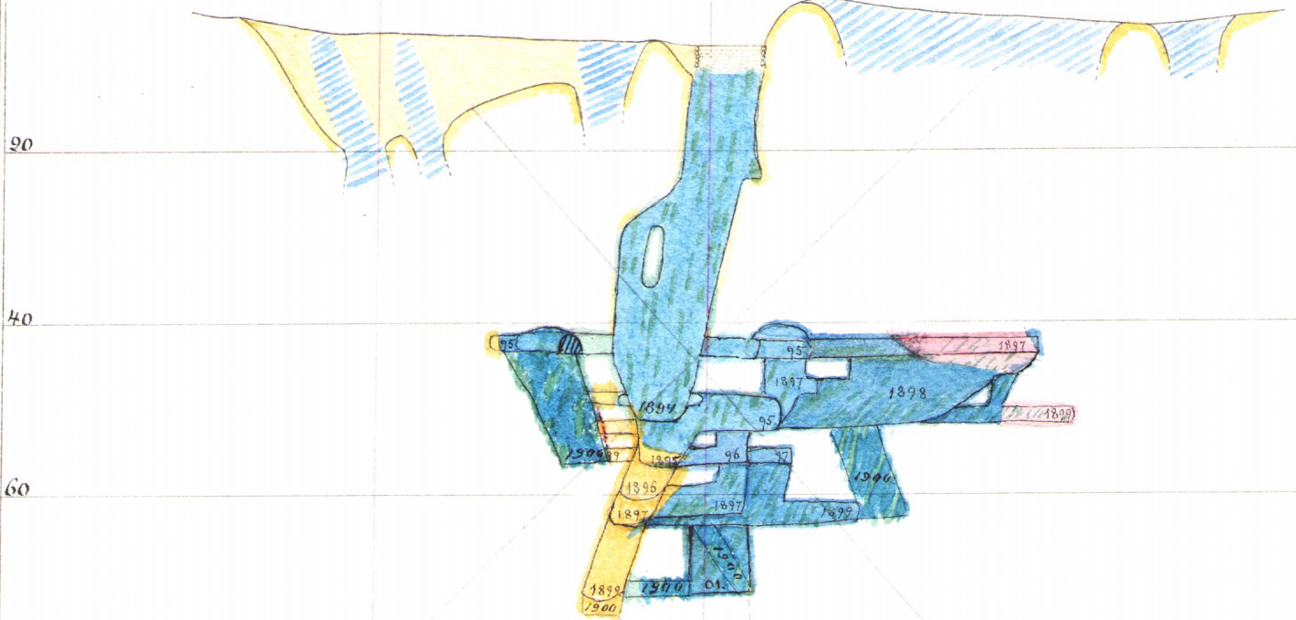
Längdprofil efter A B (Schaktet)
