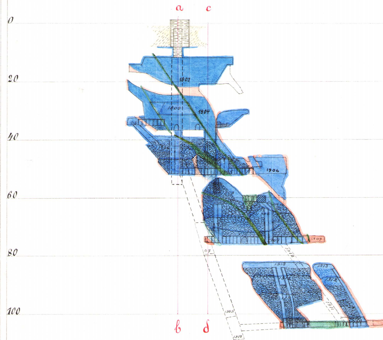
Längdprofil AB
