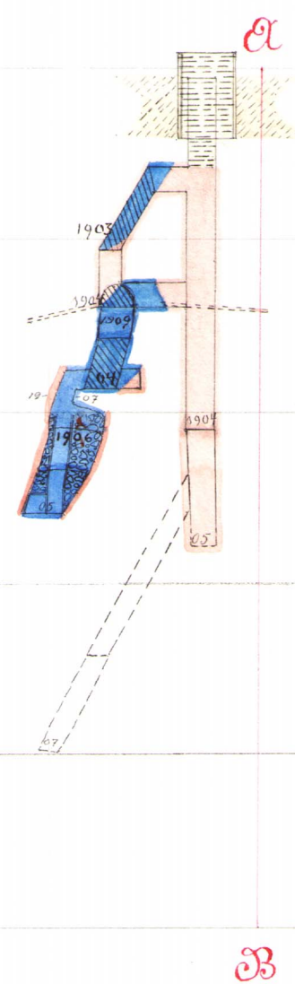
Tvärprofil a-b
