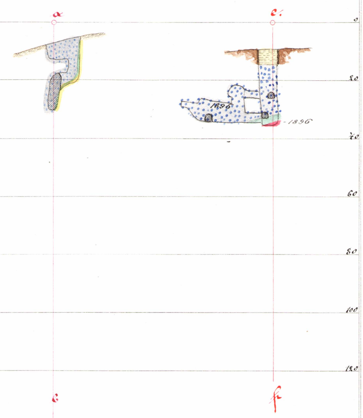
Tvärprofil efter g-h och i-k
