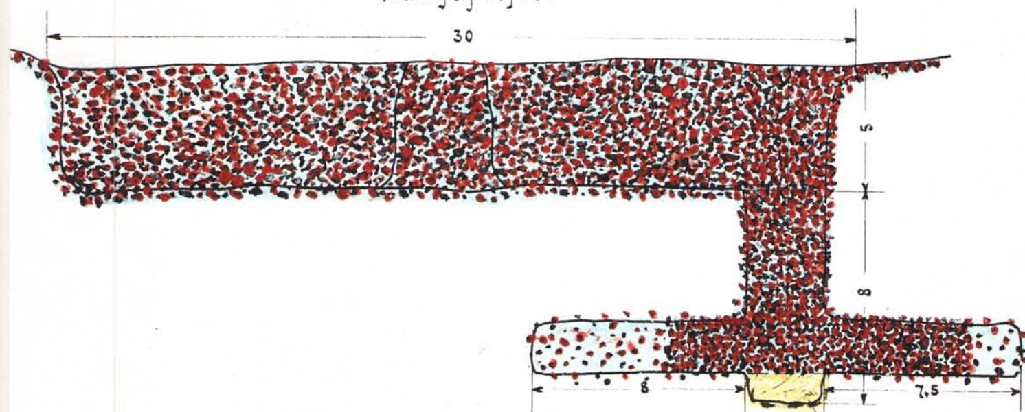
Längdprofil.
