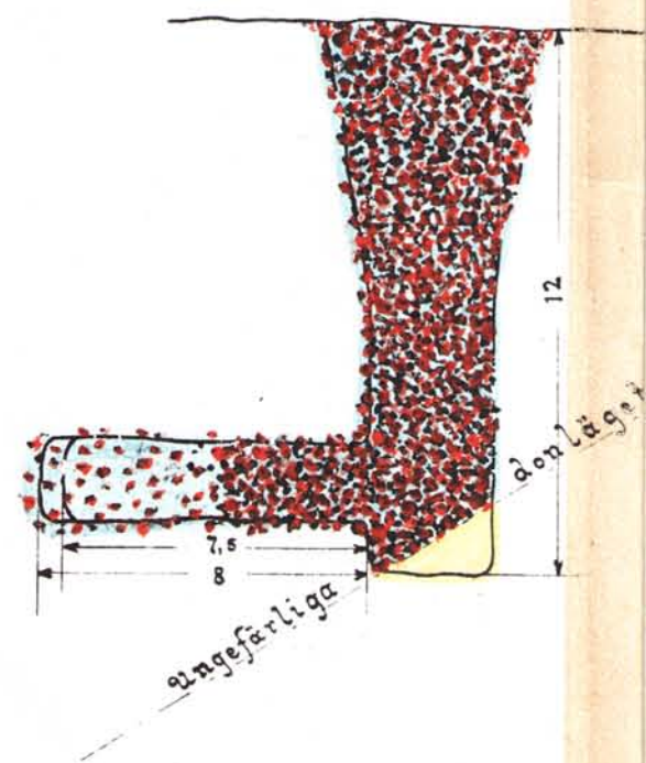
tvärprofil.
