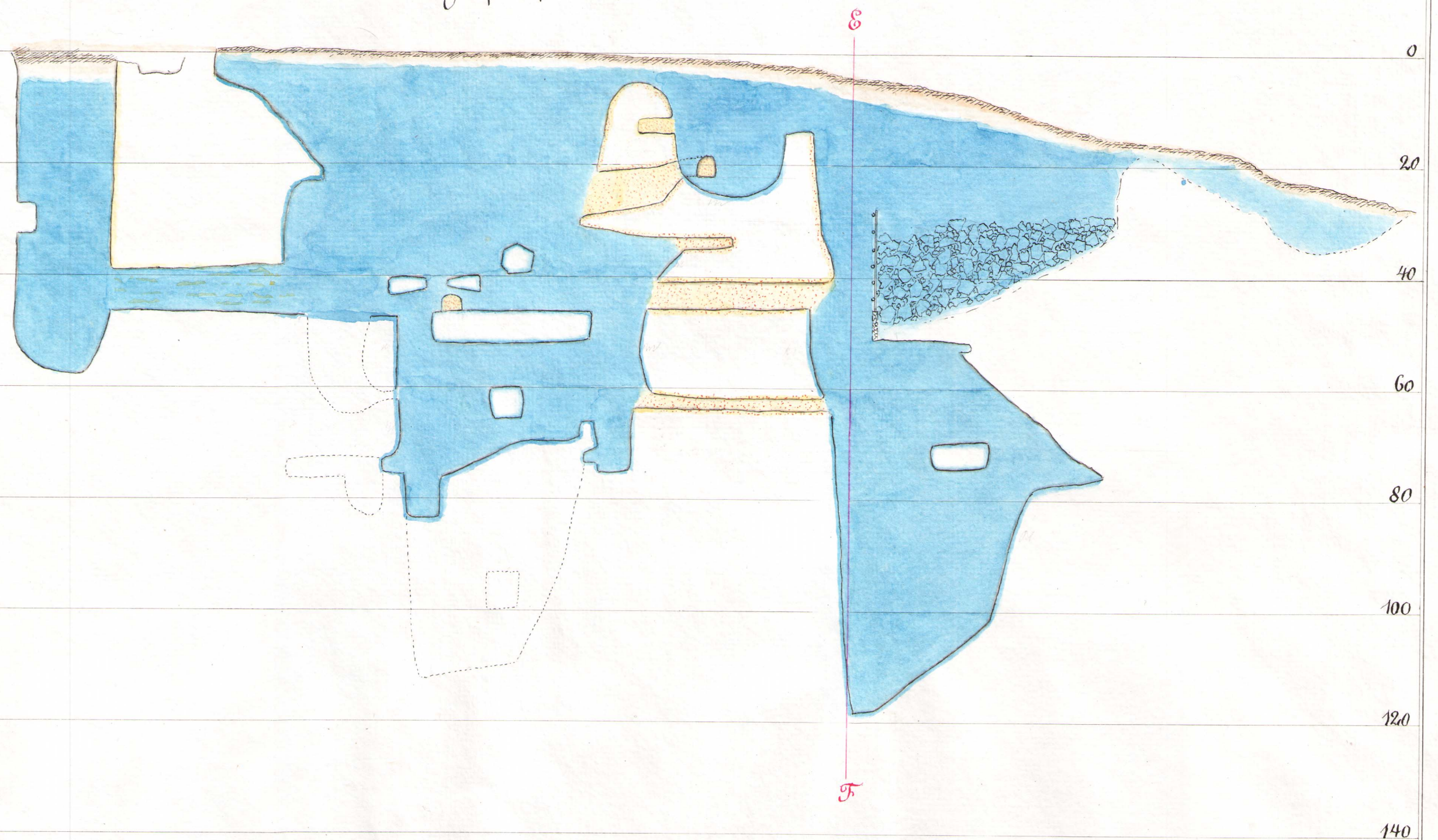
Längdprofil efter ABC
