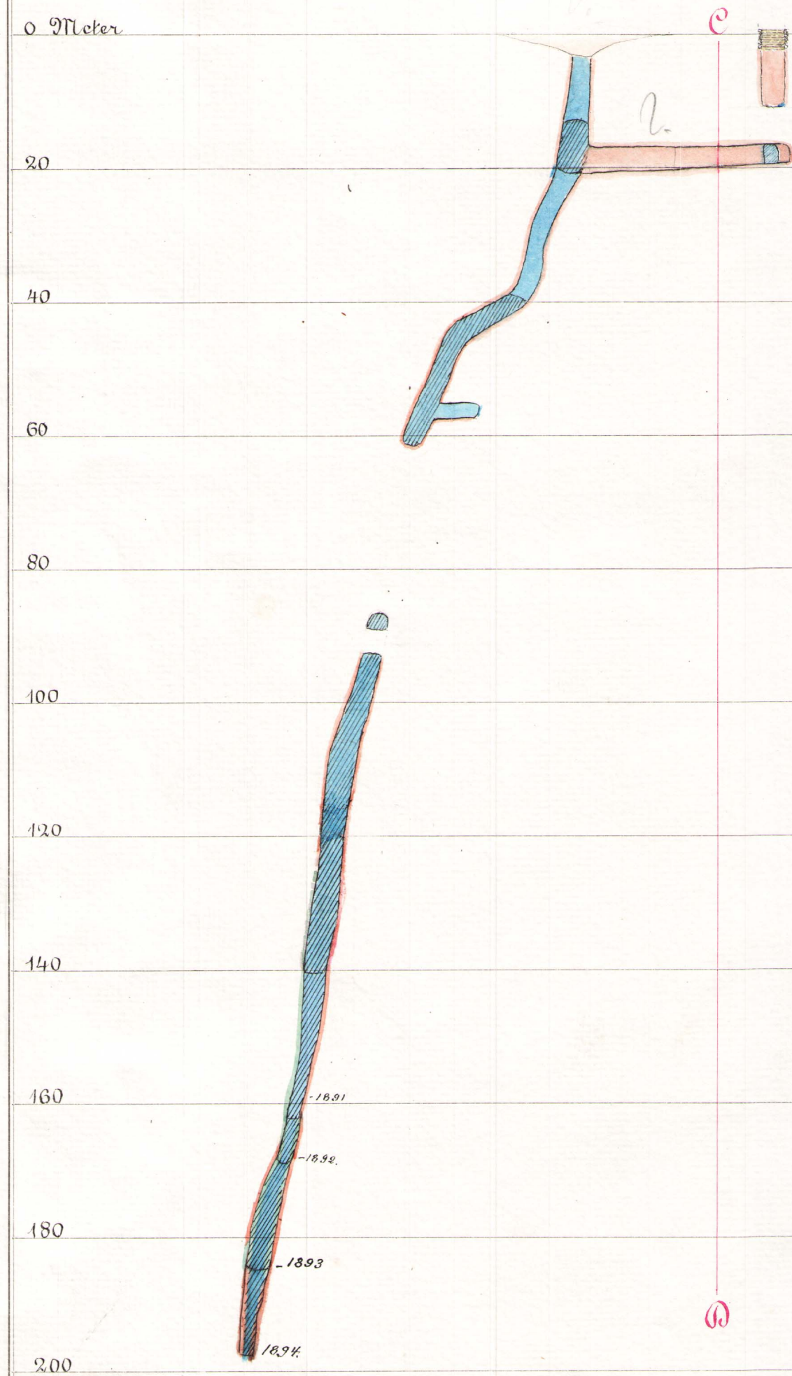
Trärprofil efter b-a
