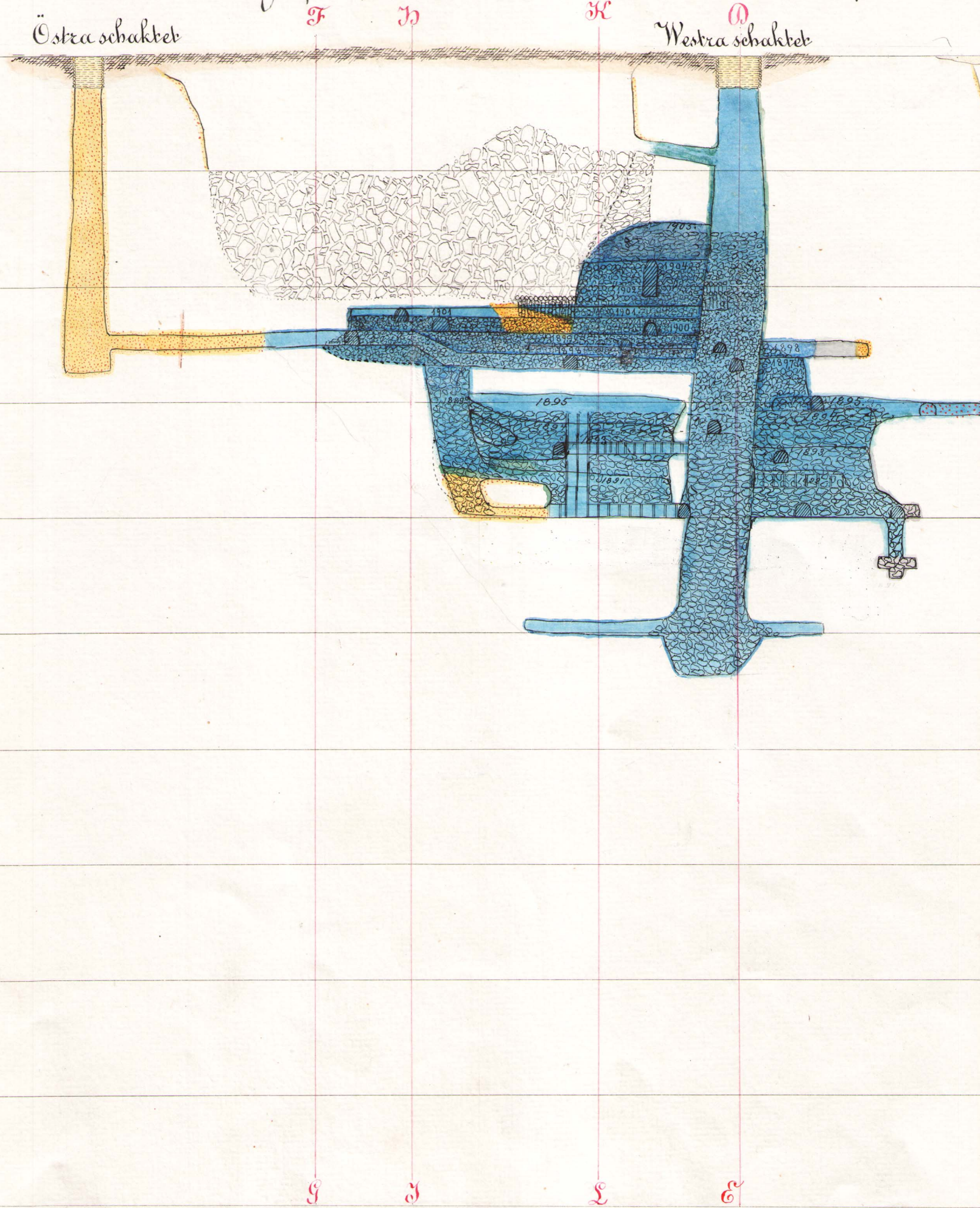
Tvärprofil efter FG
