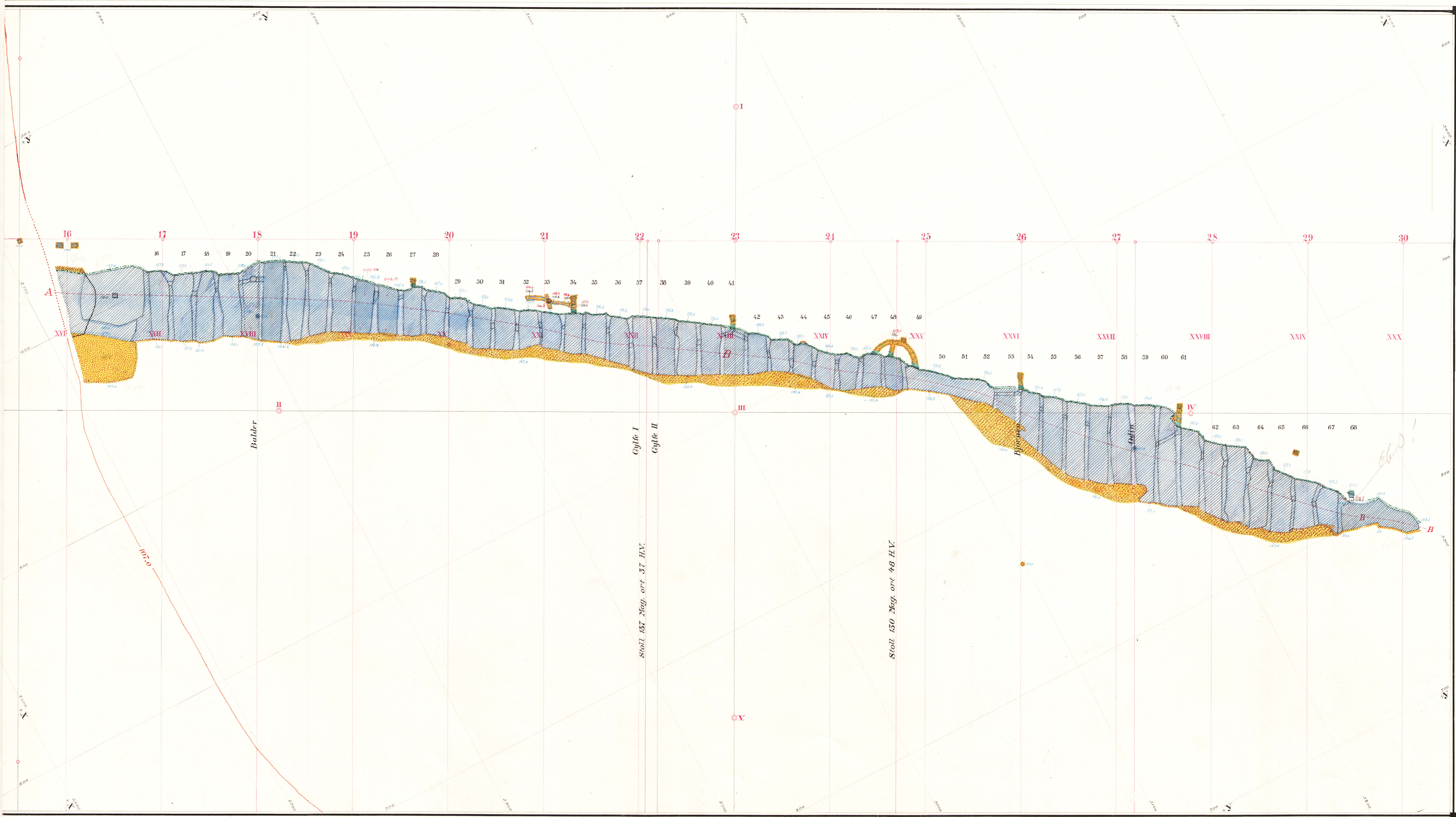
Horisontalskärning på cirka 107.0 m. nivå
