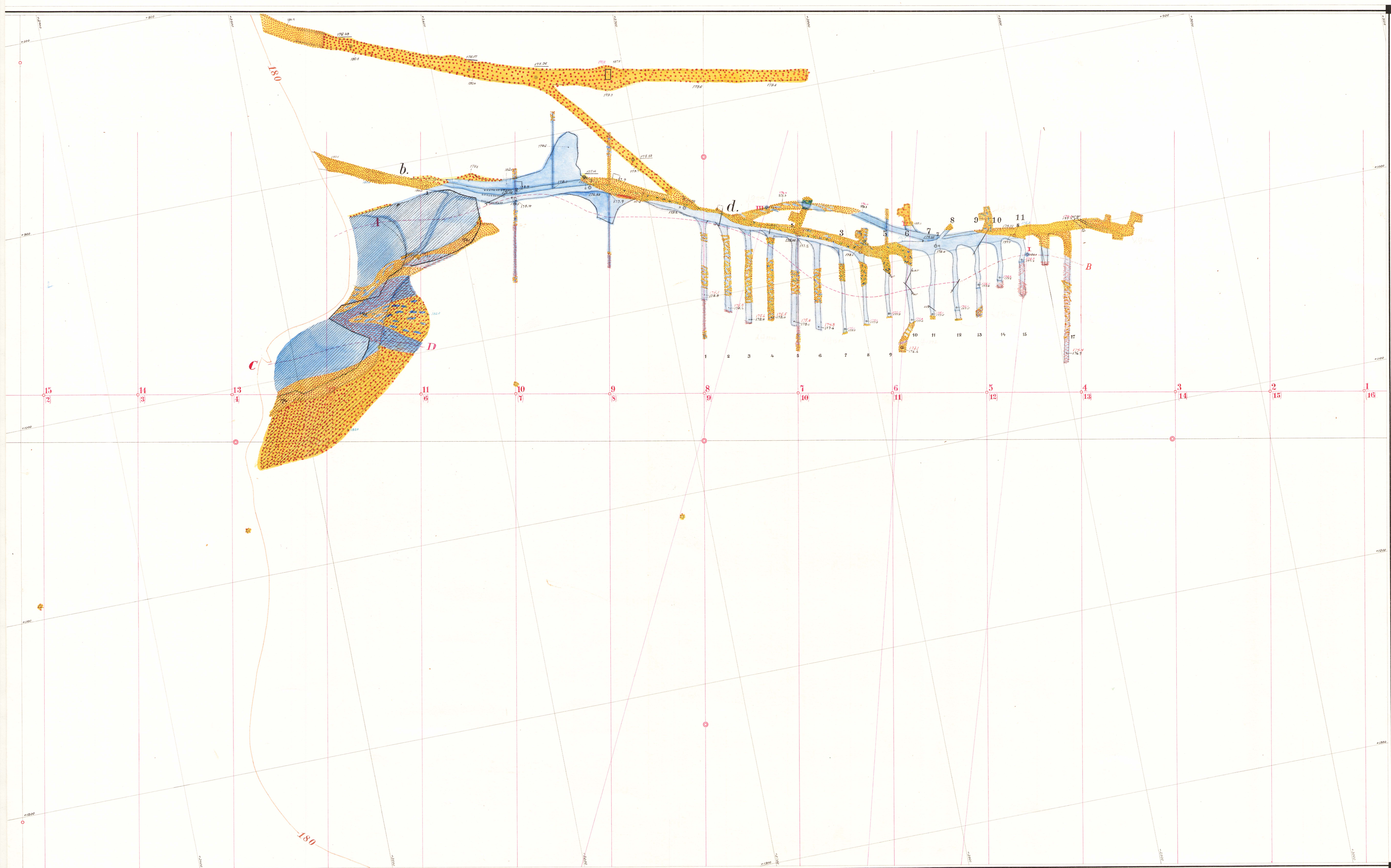
Horizontalskärning på cirka 180 m.nivå
