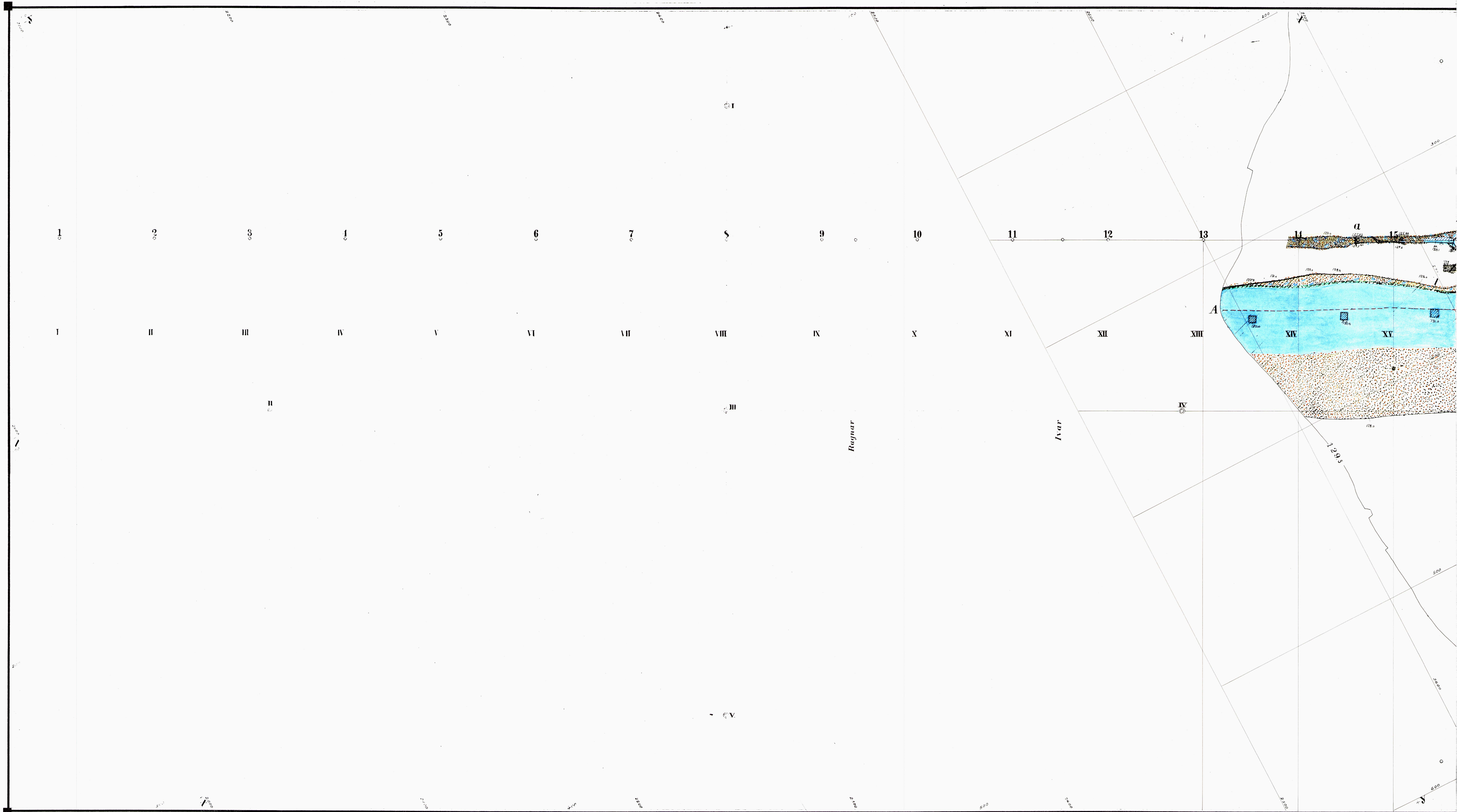
Horisontalskärning på cirka 128.0 m. nivå. Luossavaara
