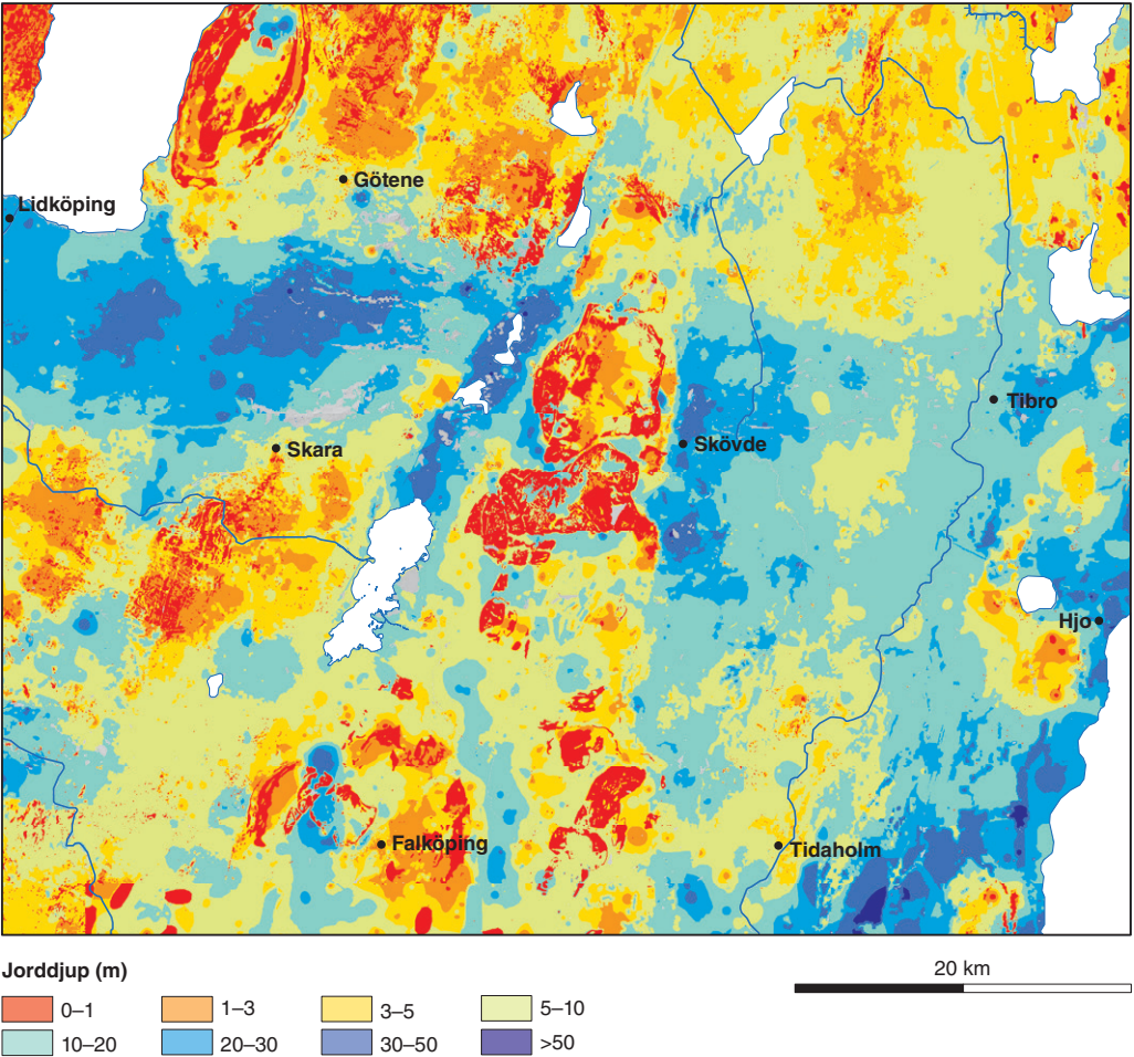
Figur 18. Översiktlig bild av jorddjupsförhållandena i regionen. De största jorddjupen finns framför allt i en zon som formats av de Mellansvenska ändmoränerna men också inom Hökensås.
