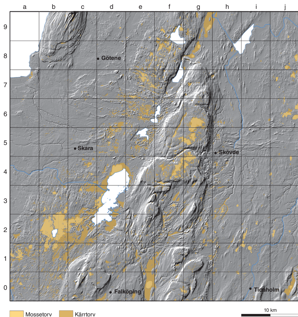
Figur 79. Utbredning av torv inom kartområdet. Peat in the mapped area.
