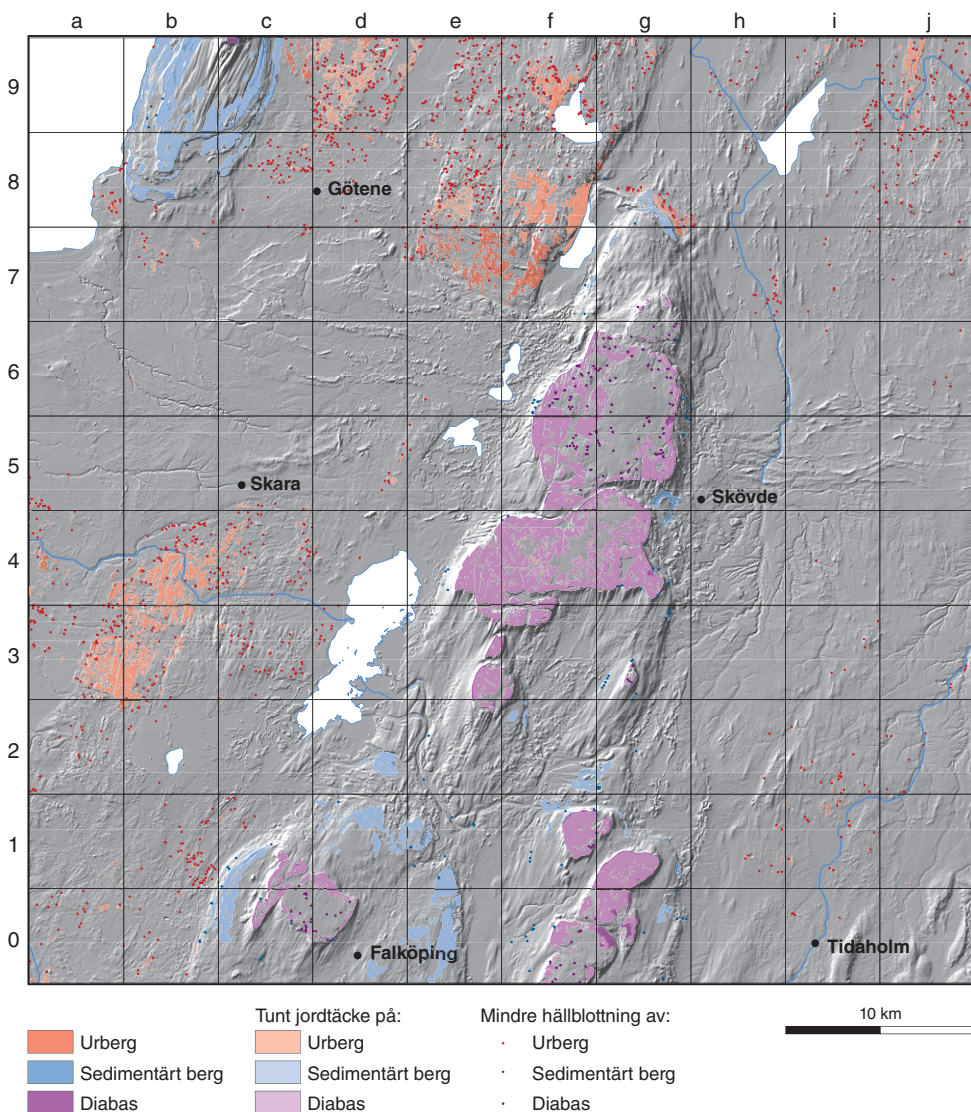
Figur 4. Förekomst av berg i dagen inom karteringsområdet.
