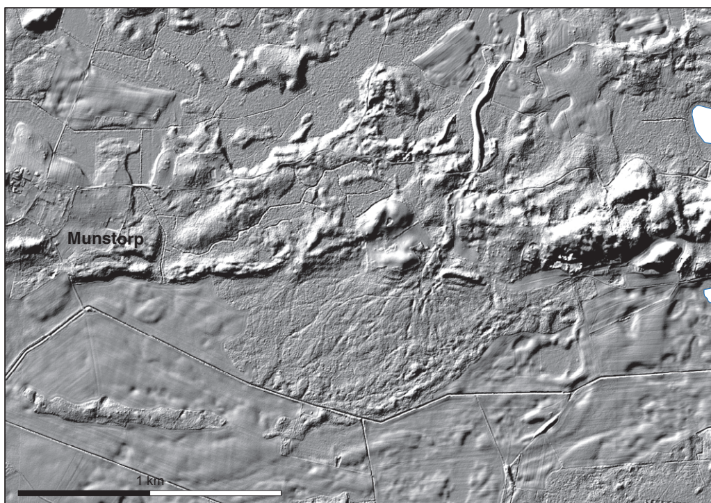
Figur 91. Sydost om Munstorp (6 d) bildades ett sandurplan vid mynningen av en ås. Denna bildning visar på ett övertygande sätt nivån för HK vid isavsmältningen. HK kan här med stor noggrannhet bestämmas till 124 m ö.h. South-east of Munstorp (6 d) a sandur has been formed at the mouth of esker drainage. This formation shows a very exact level of the highest coastline at 124 m above sea level.
