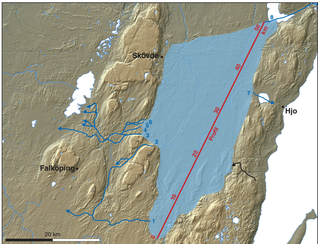
Figur 94. Områden som har varit täckta av olika stadier av Tidanissjön. Åtta av de mer betydelsefulla utloppen visas i figuren med blå pilar. Den svarta pilen visar att Vätternsänkkan under en period avvattnades ut mot väster. För en beskrivning av utloppen hänvisas till texten.
