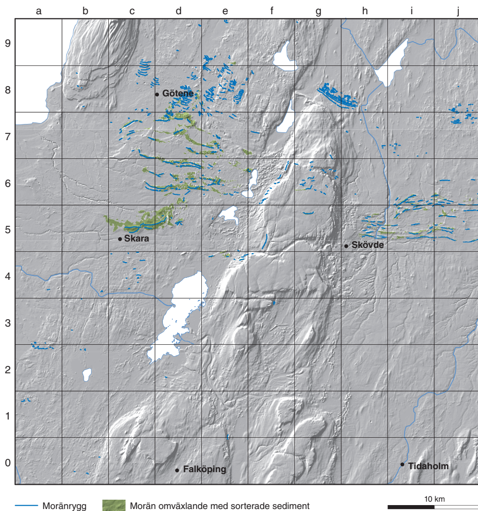
Figur 29. Randbildningar och ändmoräner i kartområdet.
