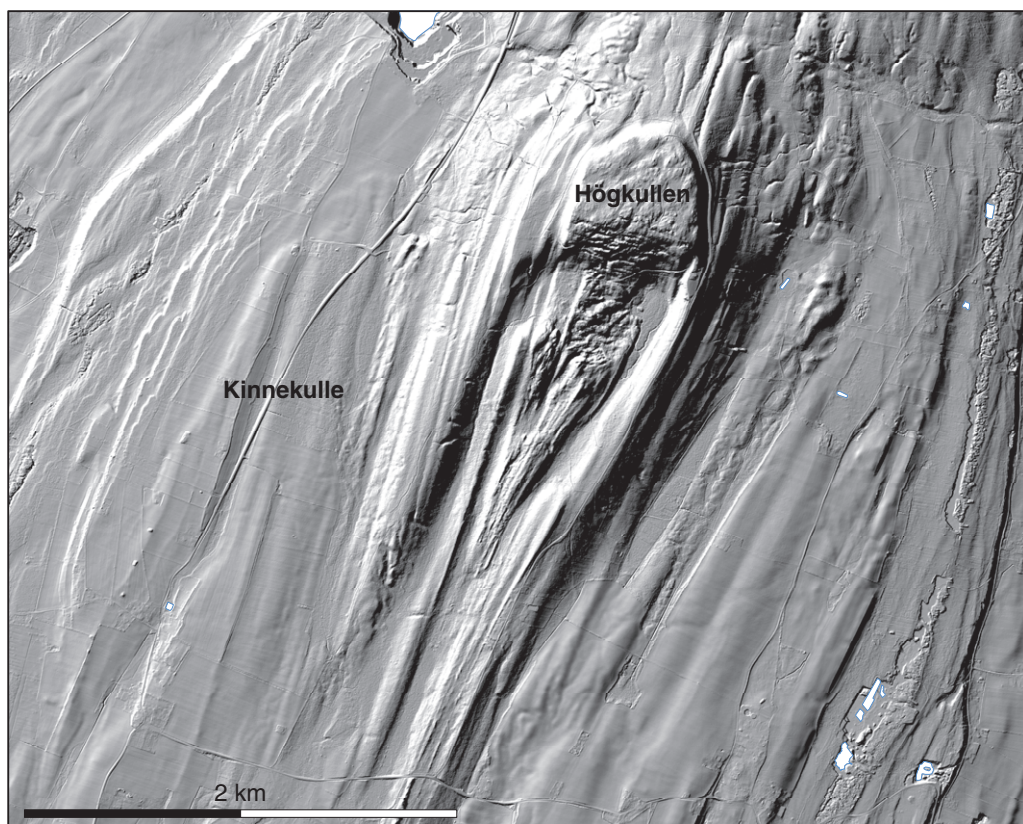
Figur 87. Svärm av drumliner på Kinnekulles övre kalkstensplatå. Söder om Höggkullen (9 c) finns en håla i drum-linsvärmen.
