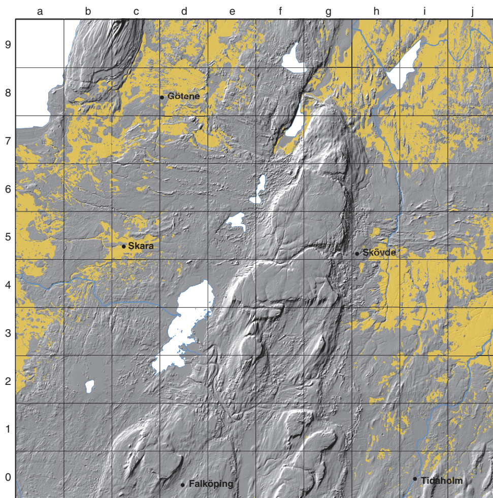
Figur 68. Lerans utbredning i ytan inom kartområdet.
