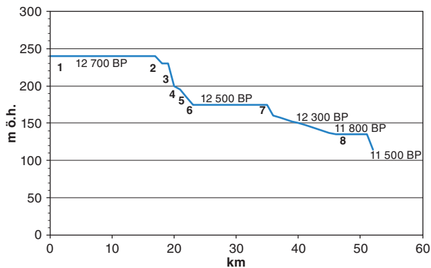
Figur 95. Tidanissjöns nivåer. X-axeln är en tänkt linje från issjöns sydligaste del upp till dess nordligaste. Utefter denna profilinje har issjöns olika nivåer ritats in. Nivåerna har uppskattats med utgångspunkt från nivåerna för de olika utloppen. Ungefärliga tider för de olika stadierna i år före nutid anges också i diagrammet.
