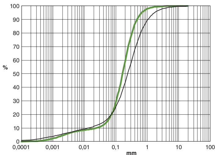
Figur 76. Kornstorleksfördelningen i flytjord som överlagrar morän vid Bjärkaskolan (3 c). Flytjorden överlagrar vindslipade block och stenar.
