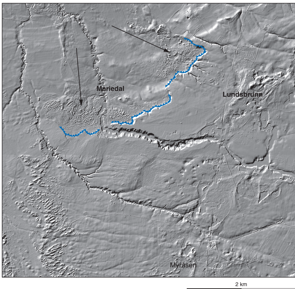
Figur 70. Skredet vid Mariedal som beskrivits av Johansson (1943) ses centralt i kartan. Pilarna pekar på det karaktäristiska mönster som bildas av skredmassorna i höjddatabasen. Skredkanten har markerats med blå linje. Landslide at Mariedal (7b–c) described by Johansson (1943) and here visualized by Lidar data.
