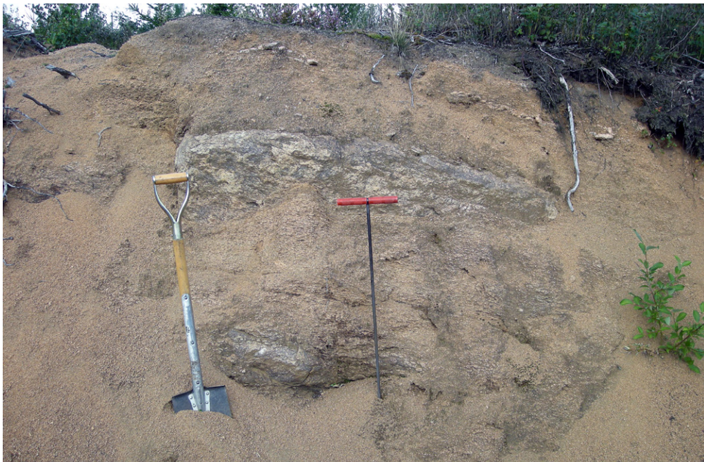
Figur 9. Täkt i vittringsgrus vid Dybergs botten. Foto: O. Larsson. Gravel pit in weathered bedrock at Dybergs botten (2a–b).
