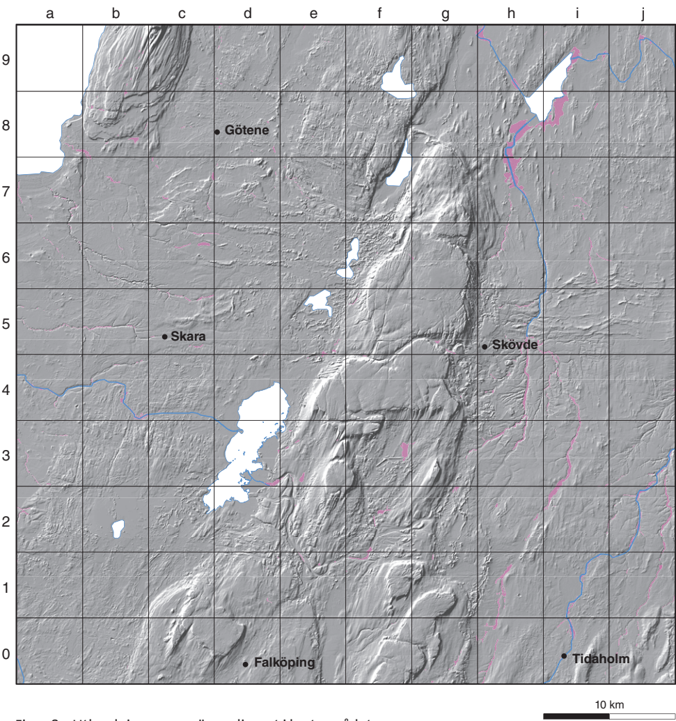
Figur 83. Utbredningen av svämsediment i kartområdet. Fluvial sediments of the mapped area.
