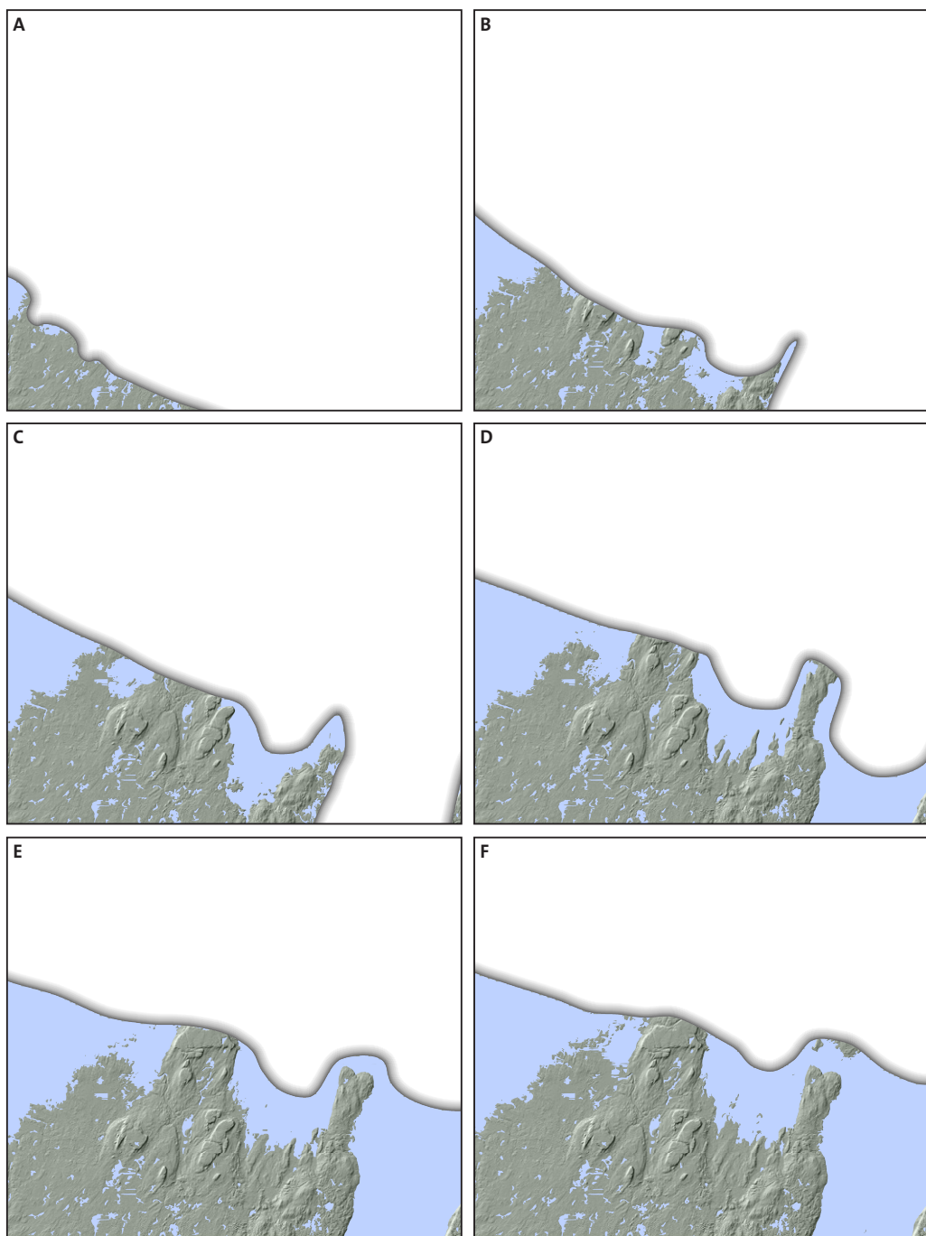
Figur 105. Områdets paleogeografiska utveckling. A. För 12 800 år sedan. B. För 12 700 år sedan. C. För 12 600 år sedan. D. För 12 500 år sedan. E. För 12 400 år sedan. F. För 12 300 år sedan.
