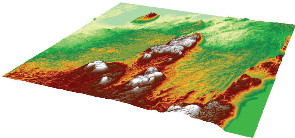
Figur 2. Denna snedbild har framställt med hjälp av Lantmäteriets höjddatabas. Vi ser på landskapet från syd-öst mot nordväst. Längst upp i bilden syns Kinnekulle vid Vänern. Längst ner i sydöstra hörnet ligger Vättern och Hökensås. De gröna områdena, uppblandade med en del gult, indikerar utbredningen av det subkambrika peneplanet. Centralt i kartbilden höjer sig platåbergen med Billingen i norr. Höjdområdet på östsidan är Hökensås, som morfologiskt har bildats som en del av det subkambrika peneplanet, men som har höjts genom tektoniska rörelser. Mellan Hökensås och platåbergen ligger en sänka som här benämns Tidansänkan. Tidan avvattnas norrut i detta lågområde. Det är i denna sänka som det bildades en issjö under isens avsmältning. Även i lågområdet i väster sker dräneringen åt norr.
