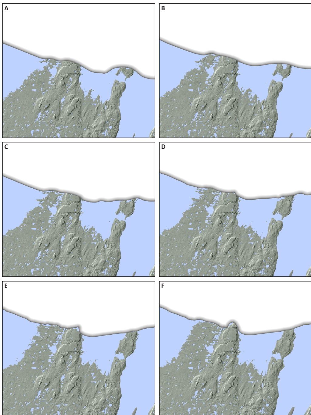
Figur 106. Områdets paleogeografiska utveckling. A. För 12 200 år sedan. B. För 12 100 år sedan. C. För 12 000 år sedan. D. För 11 900 år sedan. E. För 11 800 år sedan. F. För 11 700 år sedan.
