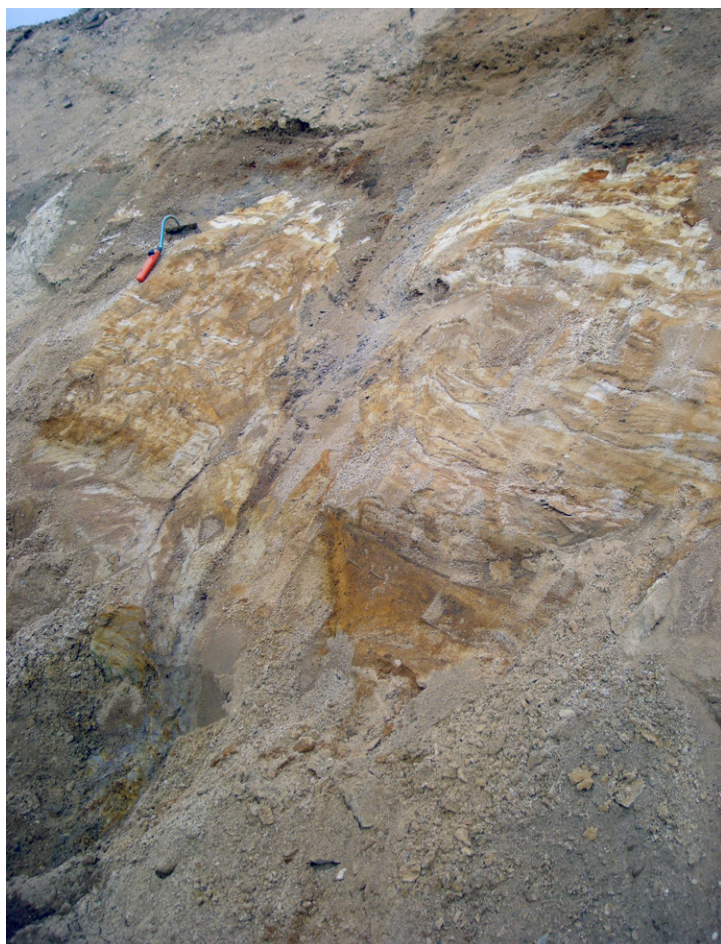
Figur 78. Fossil iskil syd- ost om Ledsjöwallen (6 d). Foto: Tore Påsse.
