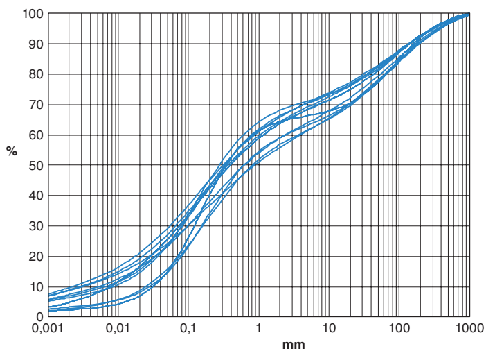
Figur 21. Prognoser som visar den totala kornfördelningen av ett antal representativa moräner inom området. Den metod som används för detta beskrivs kortfattat i texten.
