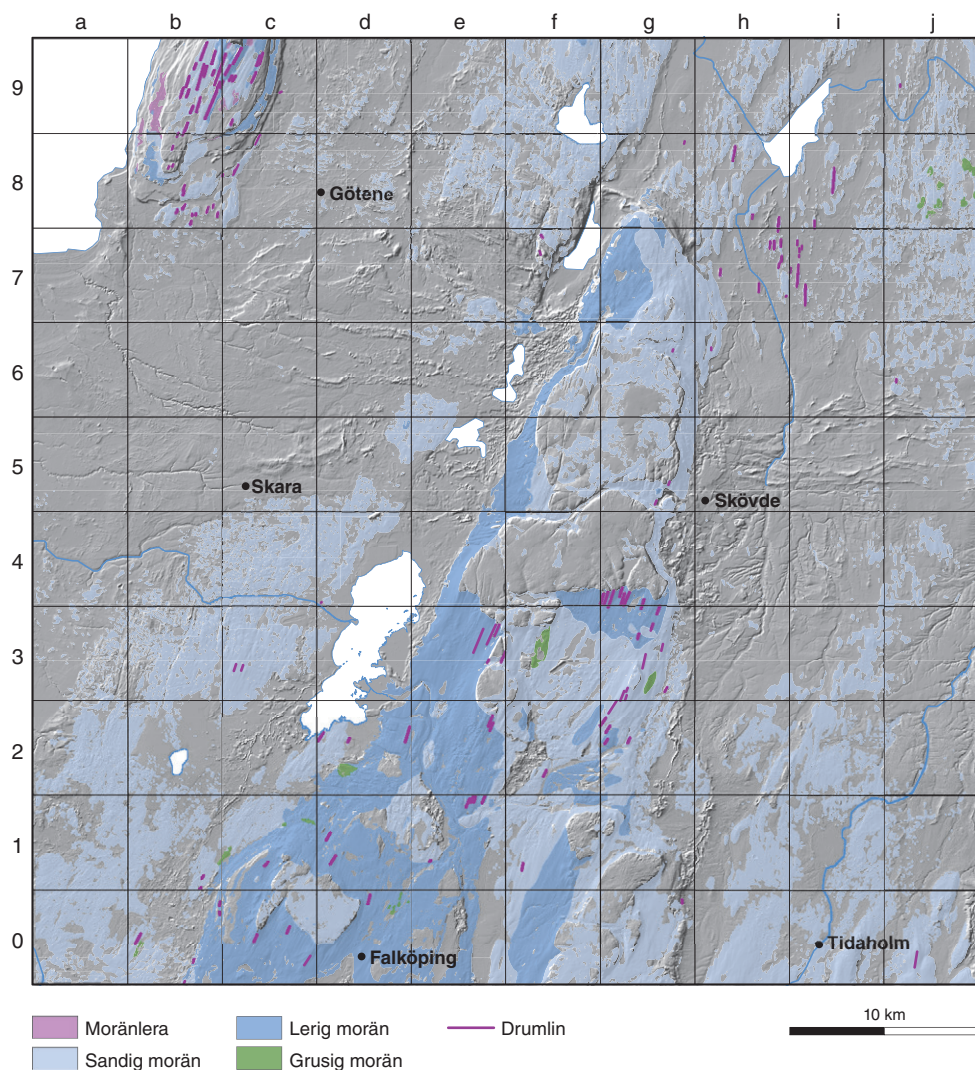
Figur 19. Moränens utbredning i ytan inom kartområdet. Ljusblå färg betecknar ytor som kartlagts som morän. Överbeteckningen L visar att moränen huvudsakligen är lerig. Lila linjer visar förekomst av stora drumliner. De mörkare blå linjerna visar var moränen bildar ryggar. Inom några få enstaka områden finns grusig morän som betecknas med grönbå färg. Morän torde finnas inom många andra områden i kartområdet, men är då täckta av yngre sediment.
