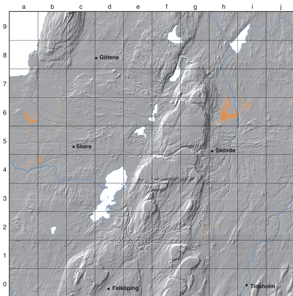
Figur 73. Utbredningen av flygsand.
