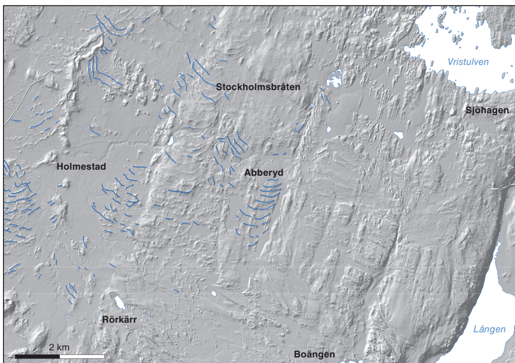
Figur 37. De Geer-moränerna framträder ofta mycket tydligt i höjddata. I denna figur syns "estuariemoränerna" vid Holmestads kyrka i den övre vänstra delen av karta. Moränryggarna vid Stockholmsbråten (8 e) syns i den centrala delen av kartan. Klyftamon ligger i kartans nederkant. Alla ryggarna är tydligt böjda.
