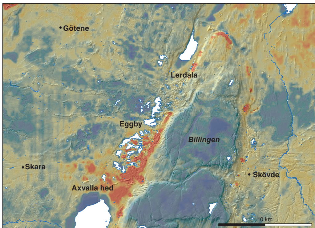
Figur 92. SGUs strålningskarta visar gammastrålningen uppmätt från flygplan. Den visar i princip innehållet av uran i berg och jord. I området är detta helt liktydigt med att det finns alunsulfider. I kartan betecknar röd färg hög strålning medan blå färg visar låg strålning. Kartan visar att tillförseln av material till uppbyggnaden av Valle härad har olika ursprung inom olika delar av formationen. I de sediment som byggt upp Axvalla hed och området norrut till Eggby finns mycket stora mängder alunsulfider. Längre norrut, söder om Lerdala, är innehållet av alunsulfider inte märkbart i strålningskartan.
