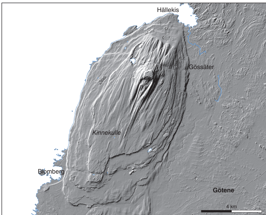
Figur 86. Svärm av drumliner på Kinnekulles övre kalkstensplatå.
