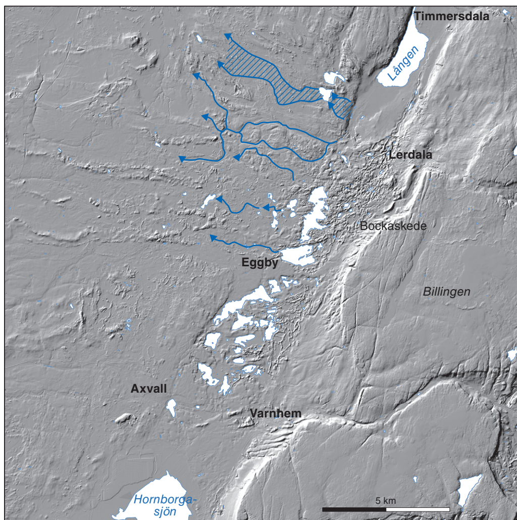
Figur 89. Höjddatabasen ger en god hjälp att analysera Valle härad. De blå pilarna visar de dräneringskanaler som successivt bildats på allt lägre nivåer när iskanten retirerade norrut. De blå rasterade ytorna visar Klyftamon, dvs. det område som kraftigt påverkades av Baltiska issjöns tappning.
