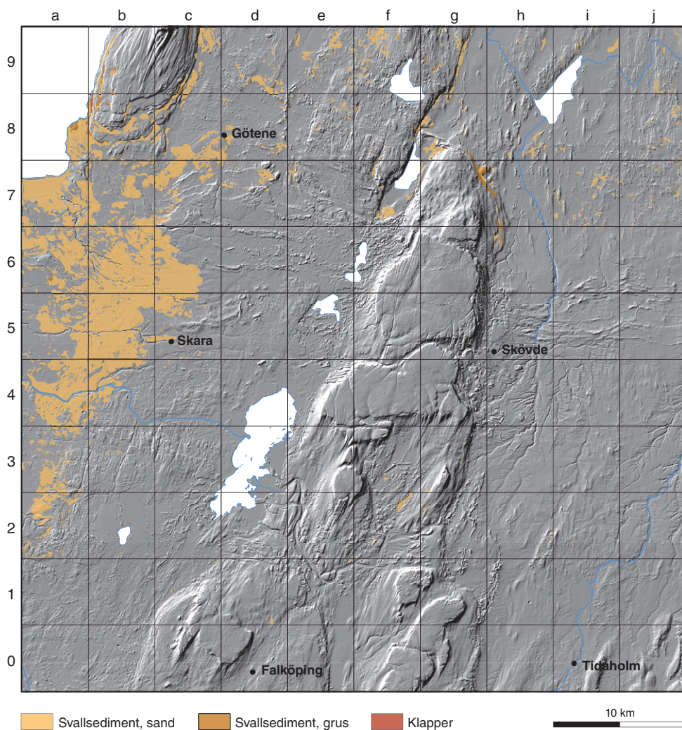
Figur 71. Utbredningen av svallsand, svallgrus och klapper. Postglacial sand and gravel in the mapped area.
