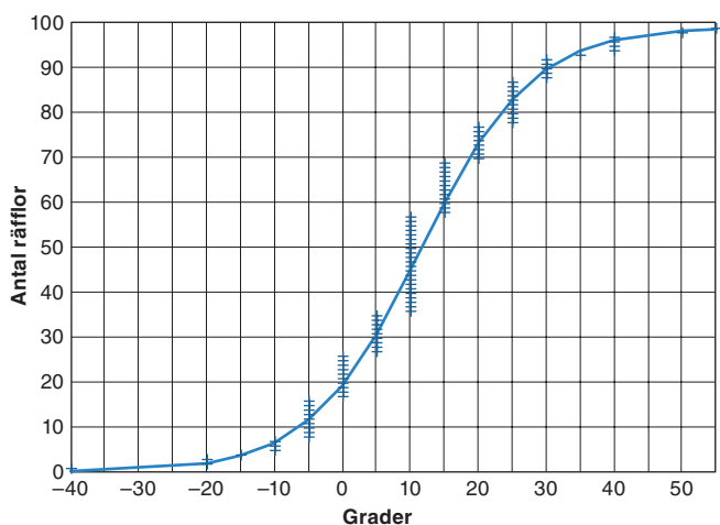
Figur 14. Statistisk analys av riktningarna på de isräfflor som påträffats vid kartläggningen. Analysen ger ett medelvärde på 10° inom kartområdet.
