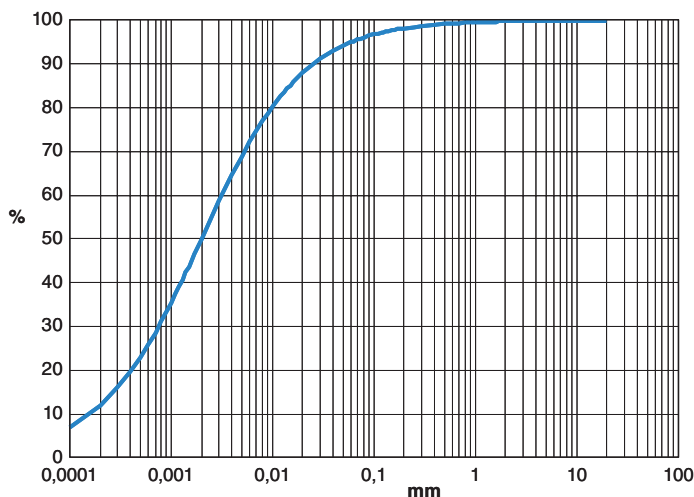
Figur 77. Valle härad är huvudsakligen uppbyggd av relativt grova isälvssediment, åtminstone i de delar där lagerföljden kunnat observeras. På ryggar i Valle härad, dvs. i sluttande terräng, förekommer ett väldigt finkornigt material i ytan. Diagrammet visar ett sådant sediment insamlat vid Slättäng (6 f). Lerhalten i detta sediment är 50 %.
