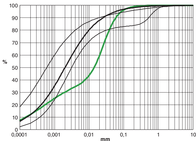
Figur 69. Kornstorleksanalyser, som har gjorts på leror från Varola (3 i), Moholm (9 j) och Götene (8 d), visas med svarta kurvor i diagrammet. Dessa tre analyser jämförs med kornfördelningen i en typisk lera från Västkusten (grön kurva). Det är anmärkningsvärt stor skillnad i kornstorleksfördelningen mellan lerorna från karteringsområdet och de från Västkusten. En tänkbar förklaring till detta ges i texten.
