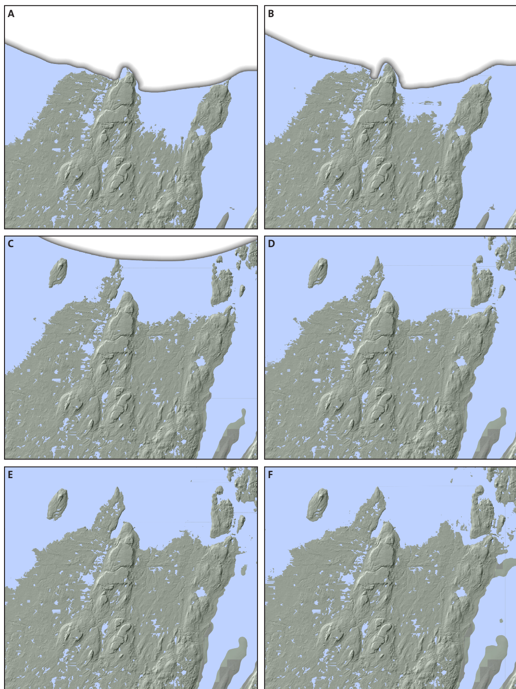
Figur 107. Områdets paleogeografiska utveckling. A. För 11 600 år sedan. B. För 11 500 år sedan. C. För 11 400 år sedan. D. För 11 300 år sedan. E. För 11 200 år sedan. F. För 11 100 år sedan.
