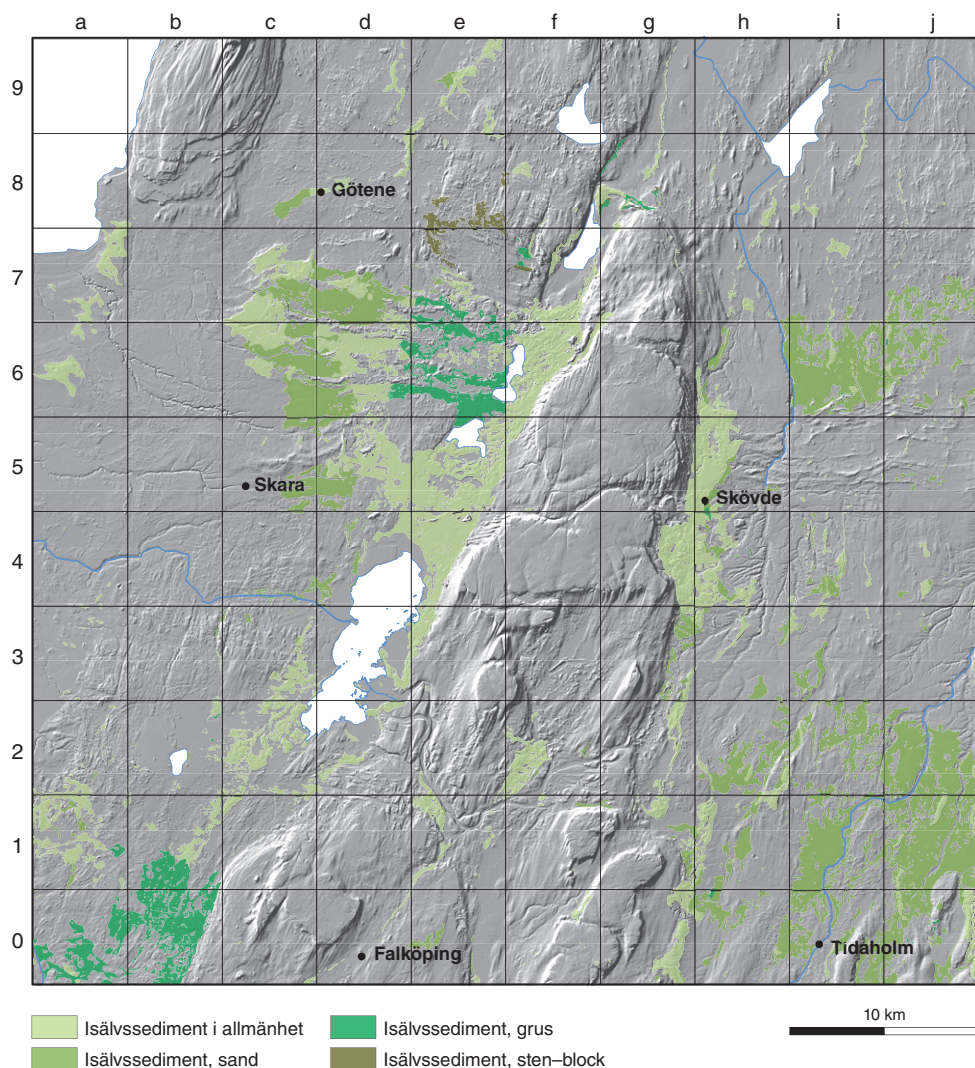
Figur 40. Utbredningen av isälvssedimenten. Sett i ett stort perspektiv förekommer det mesta av isälvssedimenten inom två kontinuerliga stråk på västra respektive östra sidan av Billingen. I kartbilden redovisas isälvssand. Denna jordart har huvudsakligen bildats i Tidanssjön och skulle därför lika gärna ha kunnat redovisas som issjösediment. Glaciofluvial deposits within the mapped area.
