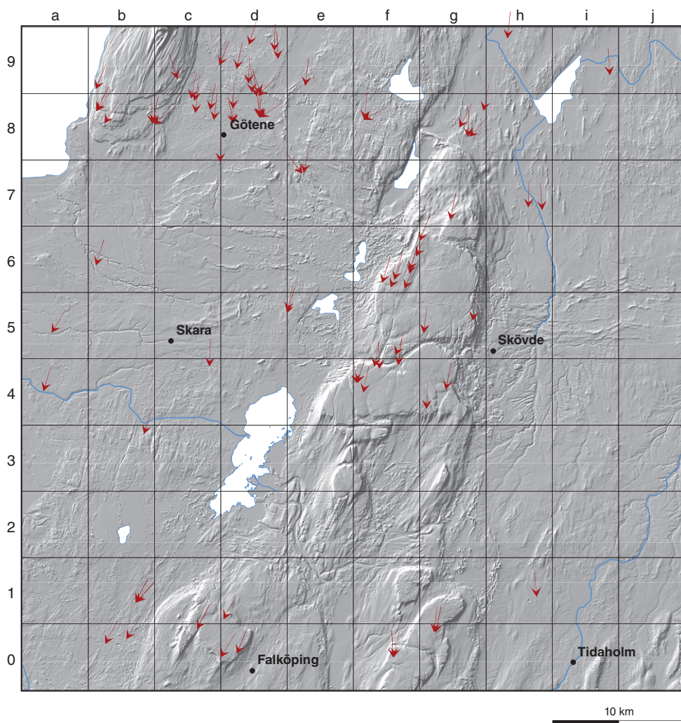
Figur 13. Förekomst av räfflor inom kartområdet. Glacial striae within the mapped area.
