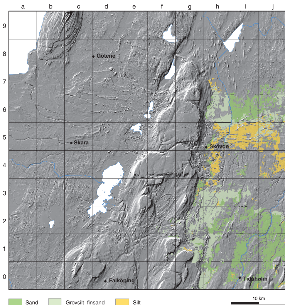
Figur 64. Utbredningen av issjösediment inom kartområdet. Glacial lake sediments within the mapped area.
