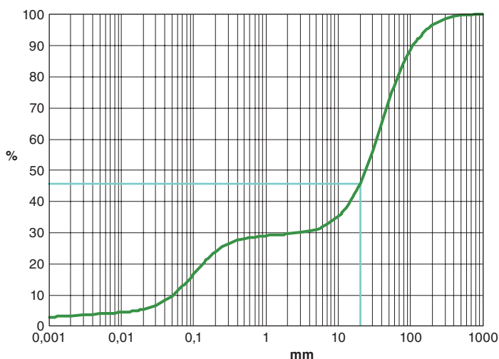
Figur 100. Kornfördelningen i den jordart som visas i de två föregående figurerna. Den del av kornfördelningskurvan som visar fördelningen <20 mm kommer från en konventionell jordartsanalys vars mätintervall har markerats med turkosa linjer. Kornfördelningskurvan >20 mm kommer från fältsiktningen.
