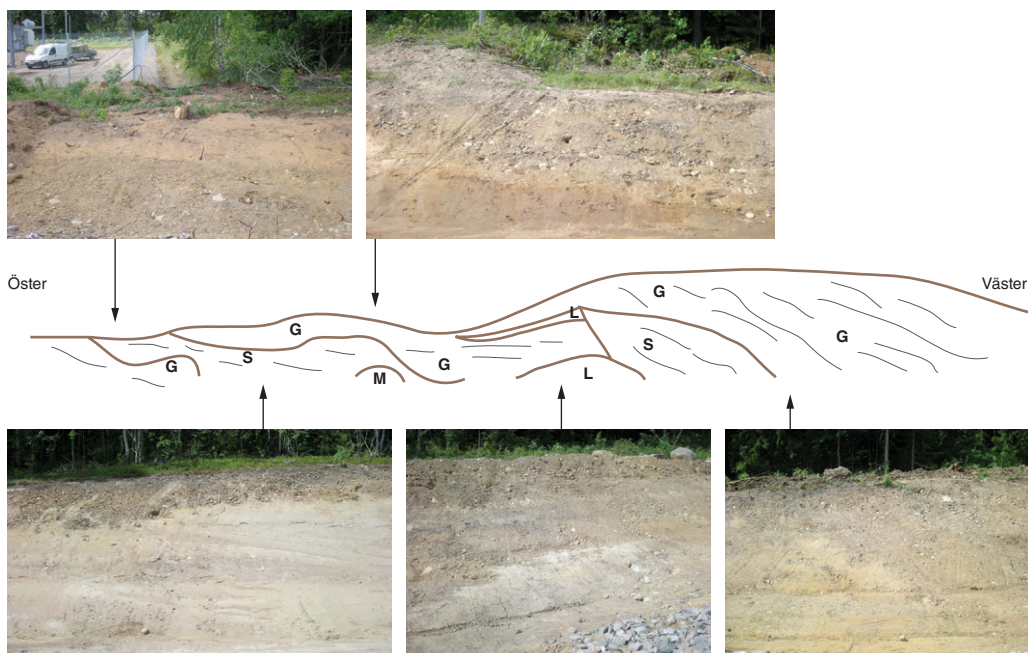
Figur 97. Skärning genom Timmersdalavallen (8 g). Under arbetet med kartan gavs möjlighet till en inblick av ryggens uppbyggnad när ett 700 m långt schakt grävdes längs med ryggen för en ny vägsträckning. Den östra halvan av denna skärning visas här. Lagerföljden består av lager som byggts upp från öster mot väster och utgörs av grovt stenigt grus (G) i botten, vilket överlagras av skiktad sand (S). I lagerföljden ingår också morän (M) och lera (L).
