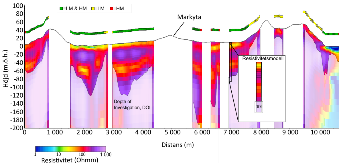
Figur 2. Exempel på resistivitssektion och resistivitsmodell samt färgkodning för LM och HM för respektive resistivitsmodell längs flyglinje.
