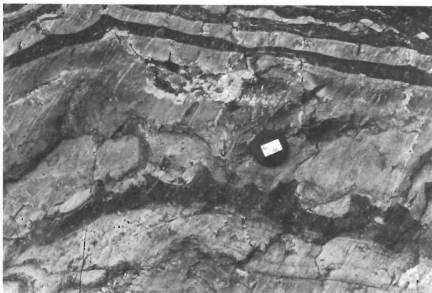
Fig. 34. "Load-casts" i kalksten visande uppåt åt NV (uppåt i bilden). Häll vid kalkbrottet 750 m N om Fanthyttan (3c), se pil i berggrundskartan.
