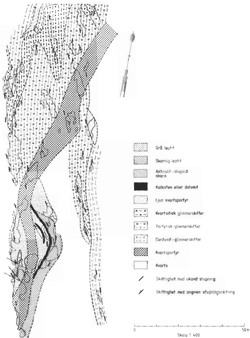
Fig. 19. Den intrusiva porfyrigången vid Lindbergstjärn (4a). Efter originalkarta av S. Ljung.
