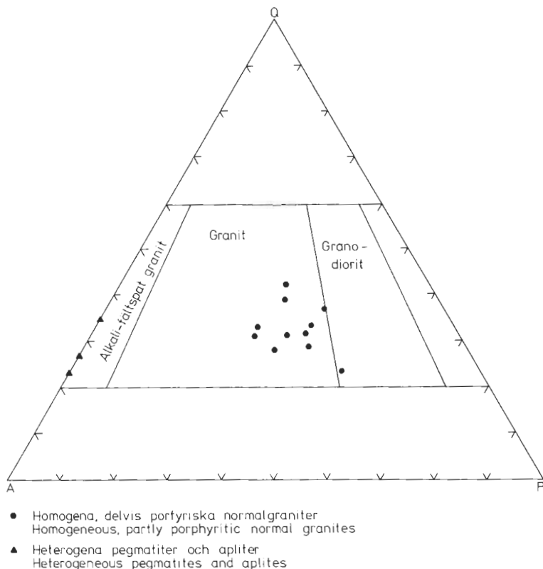
Fig. 33. De serogena intrusivbergarternas mineralfördelning.
