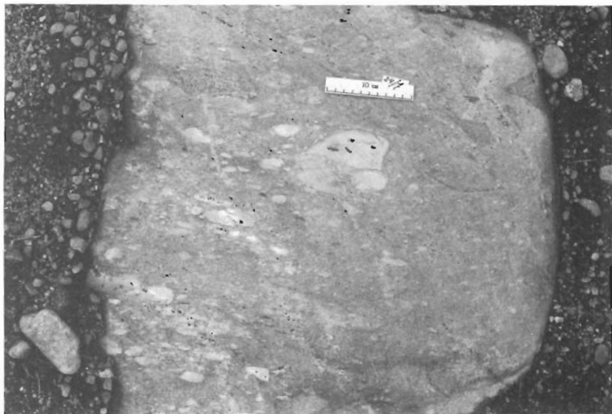
Fig. 16. Konglomerat. Häll i grustaget 2 km NNV om Nora (0b). Jfr text. Conglomerate.
