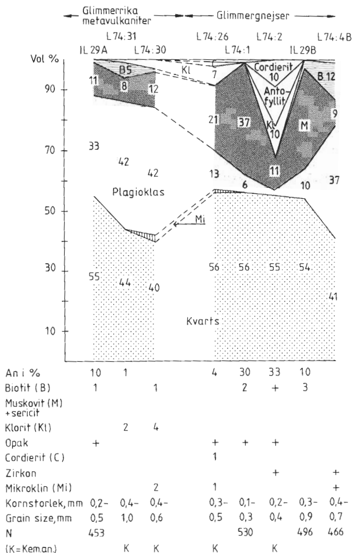
Fig. 9. Mineralfördelningen i Vasslandformationens glimmerrika metavulkaniter och glimmergnejser.
