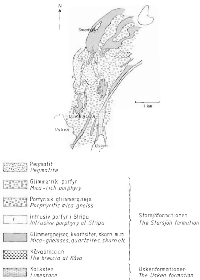
Fig. 17. Berggrunden vid Uskeboda (3b). Förenklat efter Lundberg (1971) och Ljung (1974).
