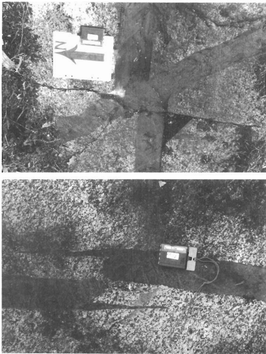
Fig. 30. Deformerade intraorogena metabasitgångar.
