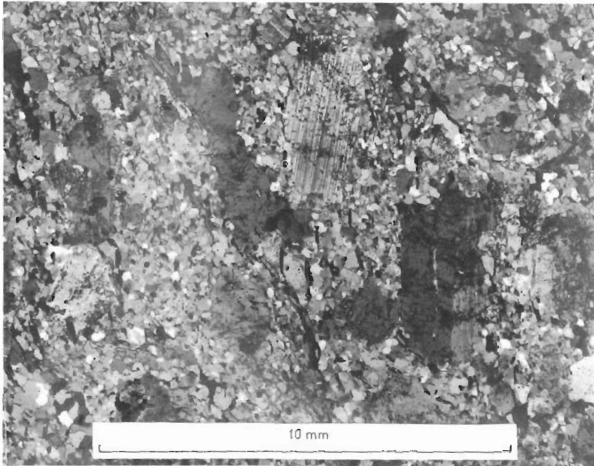
Fig. 12. Plagioklasporfyrisk metadacit ur Storsjöformationen. 1 km SO om Södermalm (1b). Halvkorsade nicoler.
