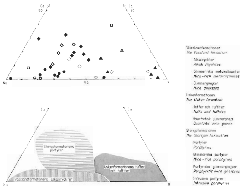
Fig. 38. Vulkaniternas och deras associerade bergarters kemiska sammansättningar, uttryckta i atomproportioner.
