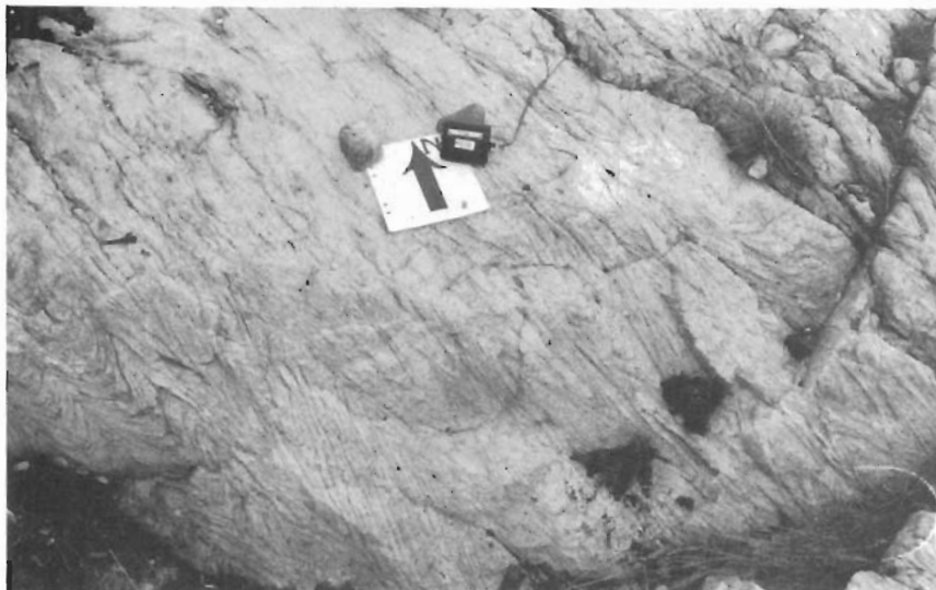
Fig. 7. Glimmerrik metavulkanit ur Vasslandformationen. 650 m NV om Kojan (0a).
