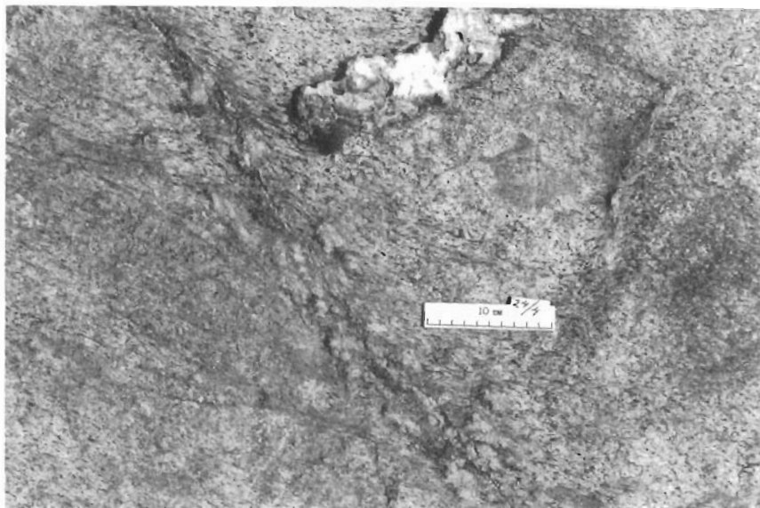
Fig. 14. Storsjöformationens glimmerrika porfyr med cordieritporfyrroblastar längs spricka. 500 m NNV om Born (0b).
