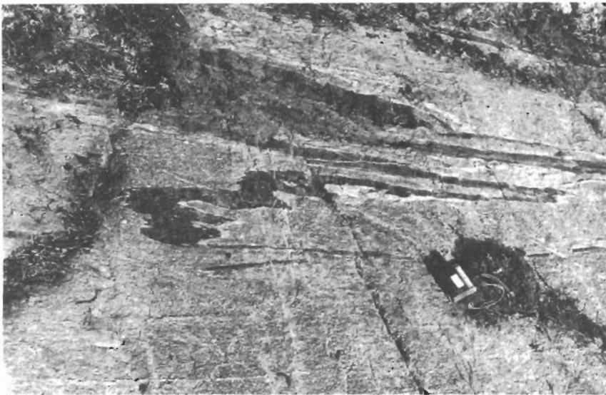
d. Metabasitgång som genom veckningen dragits in i gnejsgranitens skiffrighetsplan. 1 km V om Vedevagssjön (0d).
