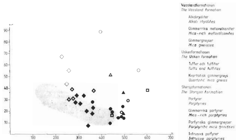
Fig. 37. Vulkaniternas och deras associerade bergarters kemiska sammansättningar, uttryckta i Niggli's t+fm - och si -värden. Normala vulkaniters sammansättningar faller vanligen inom det rasterade området (Stålhös 1969).
