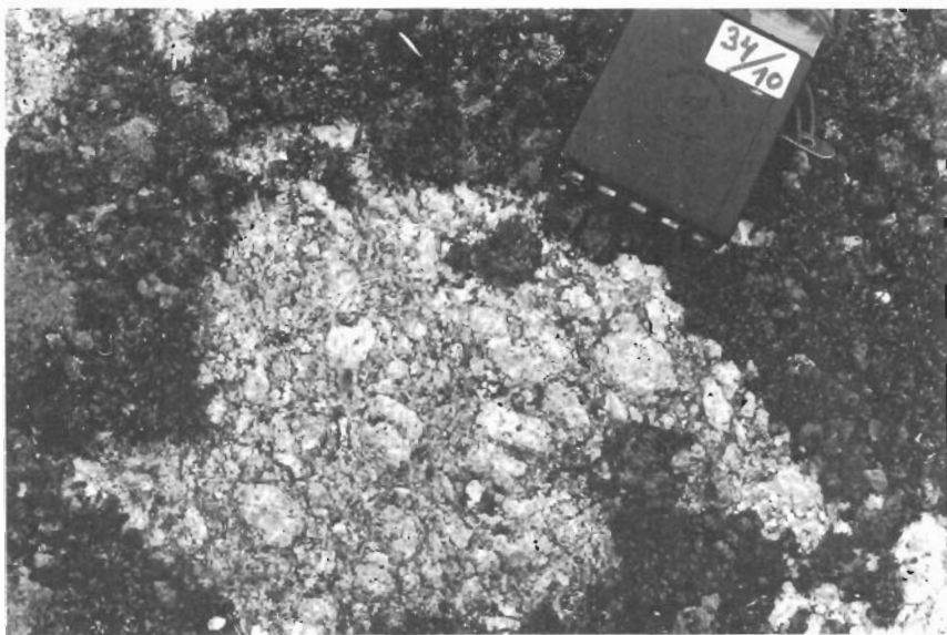
Fig. 24. Mikroklinnmegakrister av olika alder i gnejsgranit. Häll vid Anneberg (0d), 2 km Ö om Yxc.
