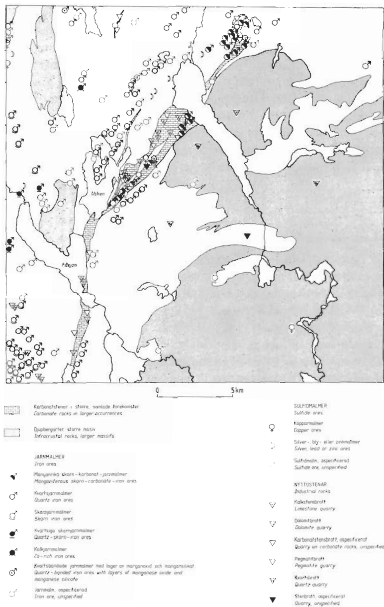
Fig. 41. Viktigare malmer och stenbrott.
