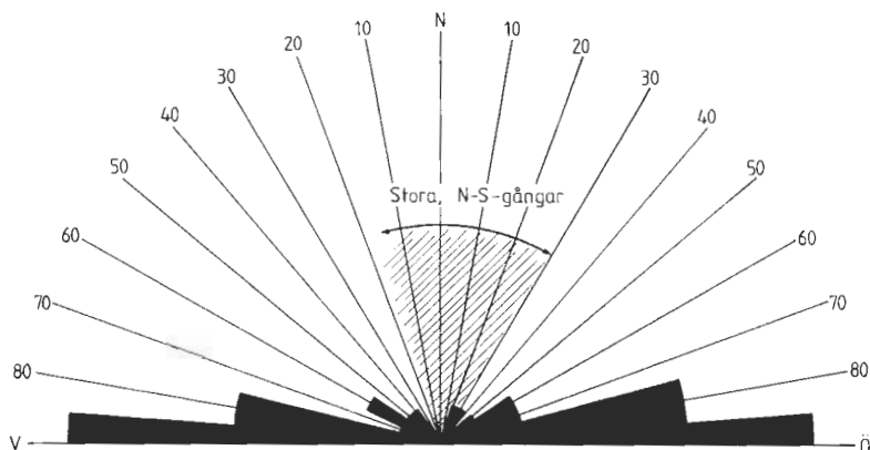
Fig. 40. Diabasgångarnas strykriktningar. N=32.
