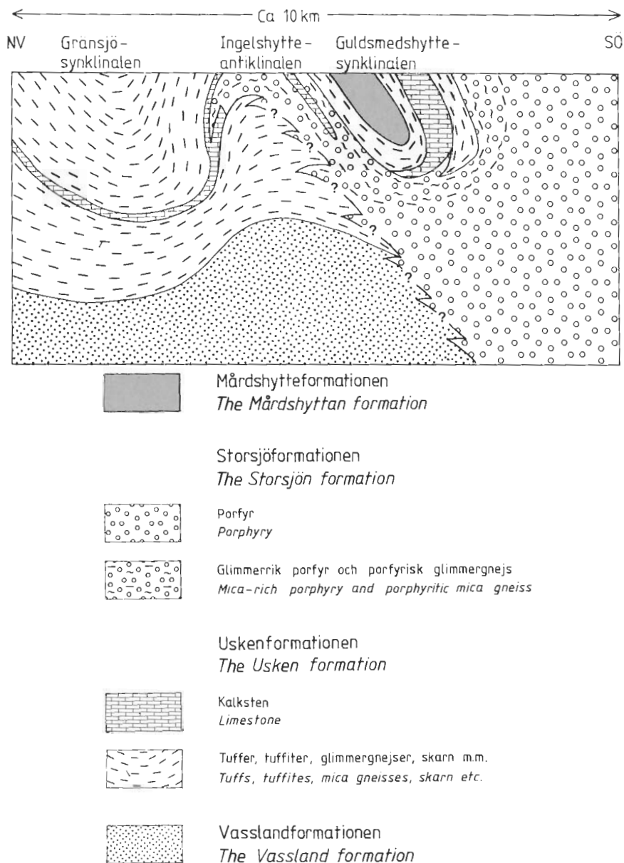
Fig. 18. Generaliserad vertikal tvärprofil genom Mårdshyttområdet (3b). Generalized profile through the Mårdshyttan area (3b).
