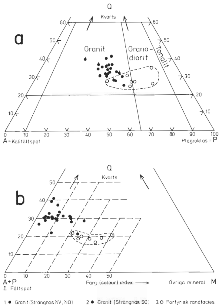
Fig. 24. Klassificering av yngre granitoider på basis av mineralogisk sammansättning enligt IUGS 1973.
