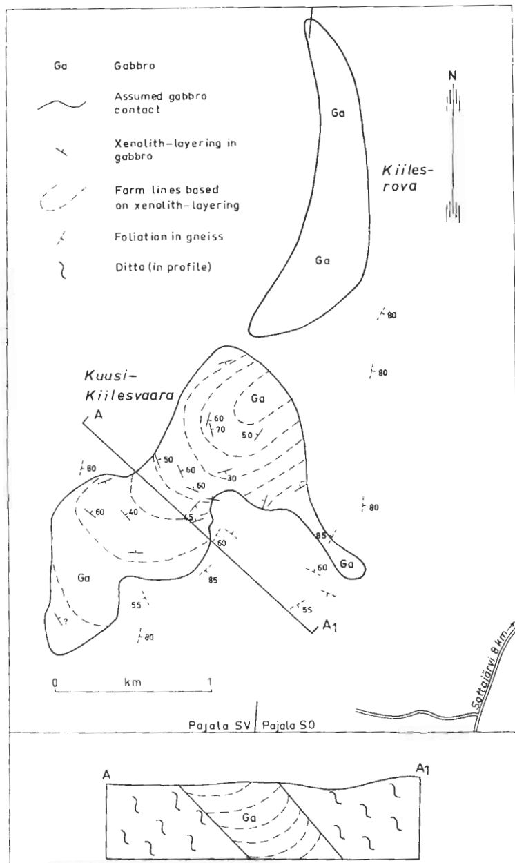
Fig. 6. The Sattajärvi gabbro showing internal structure on Kuusi-Kiilesvaara (Pajala SV-SO). Godkänd ur sekretessynpunkt för spridning. Statens lantmäteriverk 1977-04-14.
