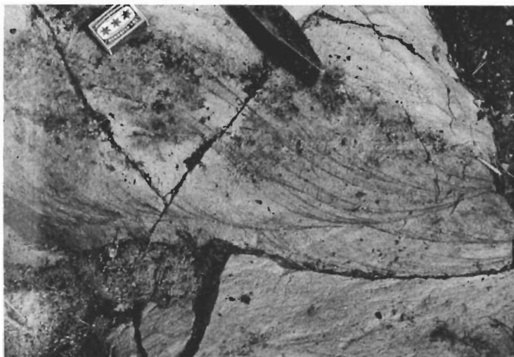
Fig. 3. Cross-bedding in quartzites of the Pahakurkkio group, Sammalvaara (Pajala NV). Diagonalskitning i kvartsit (Pahakurkkigruppen) (Pajala NV).
