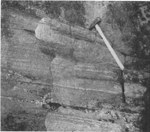
Fig. 12. Banded gneisses along Parkajoki. Bandad gnejs längs Parkajoki.
