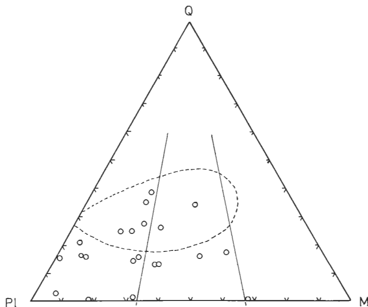
Fig. 31. Quartz-plagioclase-microcline diagram for the Jyryjoki Granite. For comparison, the area limited by a dotted line corresponds to the Lina Granite. Kvarts-plagioklas-mikrokliendiagram för Jyryjokigranit. Området inom den streckade linjen motsvarar Linagränit.
