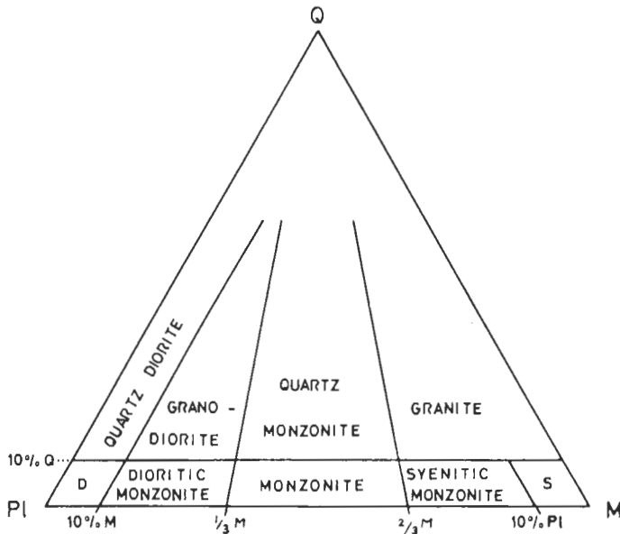
Fig. 3. Quartz-plagioclase-microcline diagram for naming rocks of acid and intermediate composition. D = diorite, S = syenite. Kvarts-plagioklas-mikrokliindigram för klassifiering av bergarter med sur och intermediär sammansättning. D = diorit, S = syenit.
