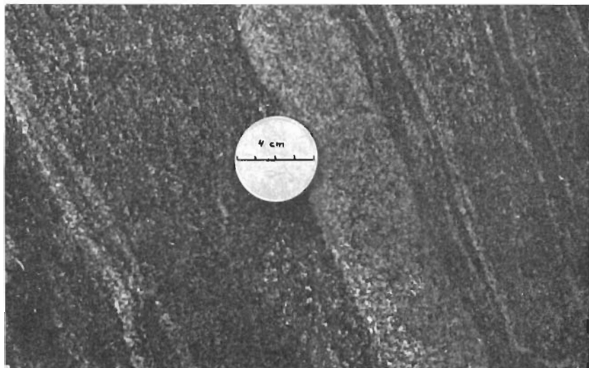
Fig. 34. Concordant to sub-concordant granitization of a biotite schist of the Haara-vaara Group, Haaraavaara. Konkordant till subkonkordant granitisation av biotitskiffer ur Haaraavaara-gruppen, Haaraavaara.
