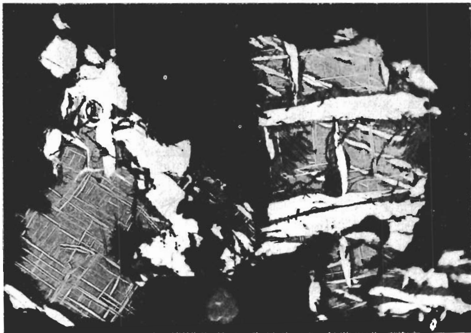
Fig. 30. Kopparmineralisering. Bornit (grå) med lameller och listformade korn av kopparkis (vit). Mörkgrå, smala sliror i bornit och kopparkis utgörs av covellin, som även omger kopparkislamellerna. Svart = kvarts. Gruvberget, borrhål 61103, 110.1 m. Polerprov. Vanl. ljus, \times 450 , immersion.
