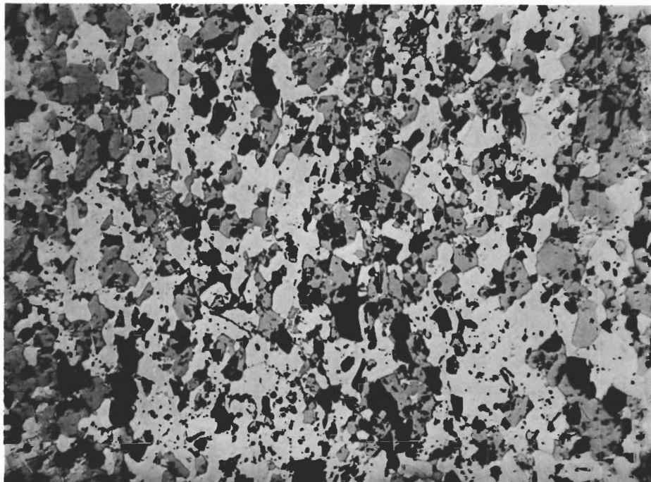
Fig. 51. Magnetitrik blodsten. Korn av magnetit (ljusgrå) i hämatit (gråvit). Svarta korn utgörs av kvarts och apatit. N om Storgruverymningen. Polerprov. Vanl. ljus, \times 75 . Magnetite-rich hematite ore. Magnetite grains (light grey) in hematite (grey white). Black grains are quartz and apatite. N of Storgruverymningen. Polished section. Ord. light, \times 75 .
