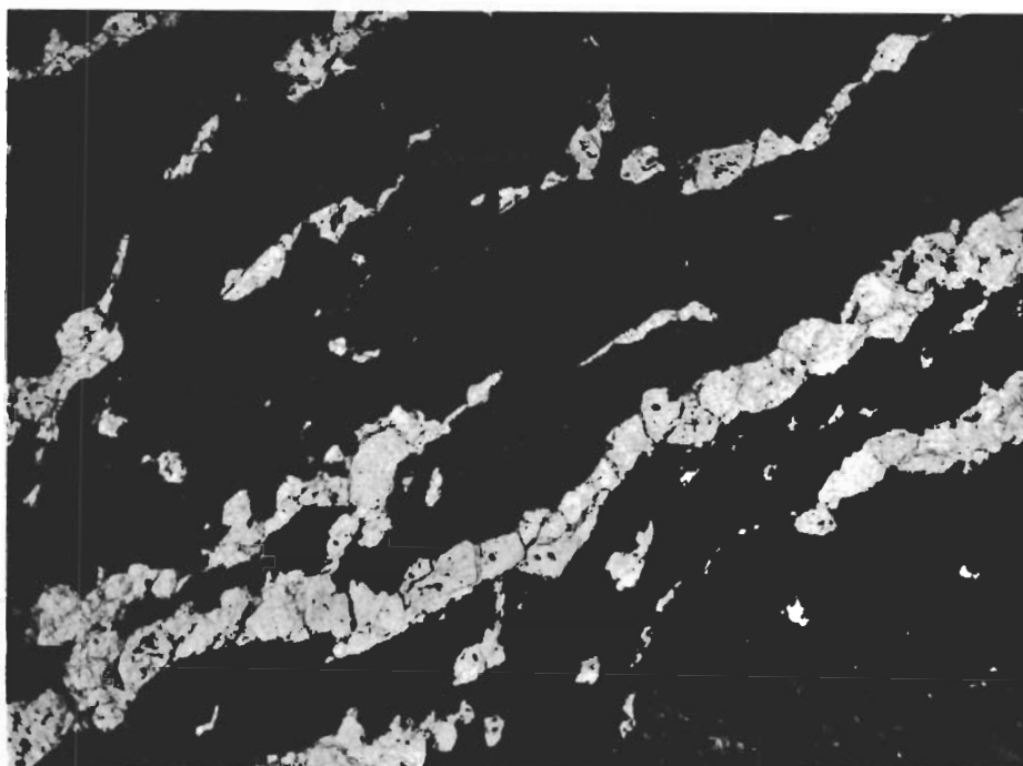
Fig. 48. Apatitslirig blodsten. Hämatit = svart. Apatit = gråvit. I nedre, högra hörnet ett granatkorn (svart med gråsvarta fläckar). Gruvberget, borrhål 23, 15.1 m. Slipprov. Vanl. ljus, \times 40 .
