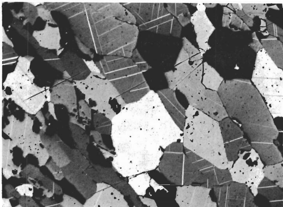
Fig. 46. Fintjällig, parallellstruerad blodsten. Hämatit = vit till mörkgrå. Svarta korn mellan hämatiten utgörs av apatit. Gruvberget, borrhål 58101, 93.8 m. Polerprov. Nic. +, \times 88 . Fine-grained hematite ore with parallel texture. Hematite = white to dark grey. Black grains between the hematite are apatite. Gruvberget, drill-hole 58101, 93.8 m. Polished section. Nic. +, \times 88 .
