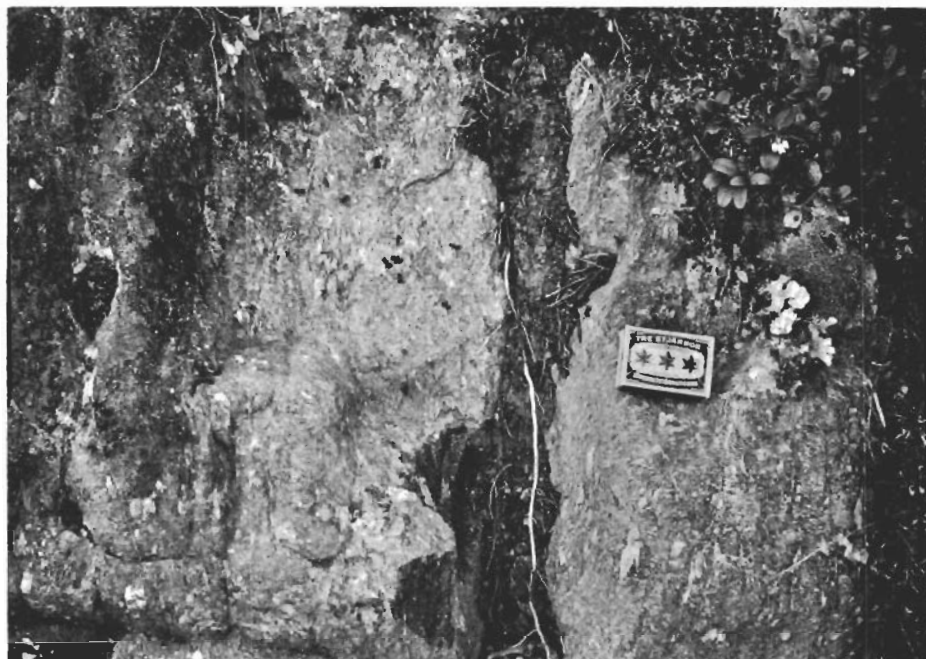
Fig. 4. Albitporfyr. Östra delen av Bergsmannivaara. Albite porphyrite. Eastern part of Bergsmannivaara.
