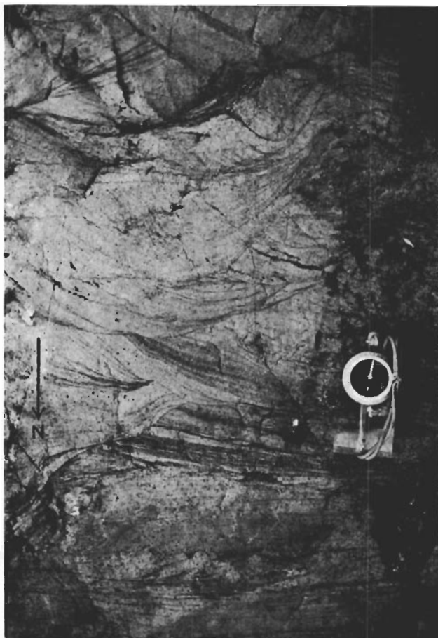
Fig. 7. Diagonalskiktning i kvartsitsandsten. SÖ om Pikku Luongasjärvi. Cross-bedding in quartzitic sandstone. SE of Pikku Luongasjärvi.
