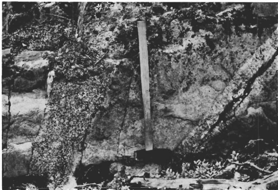
Fig. 10. Kvartsitsandsten genomsatt av granodiorit (till vänster) och Linagranit (till höger). Kiilavaara.
