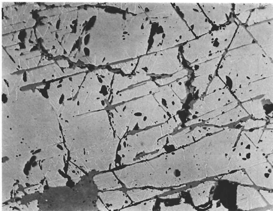
Fig. 80. Magnetit (grå) med titanit (mörkgrå; dels lameller, dels sliror; i nedre vänstra hörnet ett större aggregat) och hämatit (gråvita, smala lameller). Svart = håligheter i provet. Tansari, borrhål 60403, 36.2 m. Polerprov. Vanl. ljus, \times 185 .
