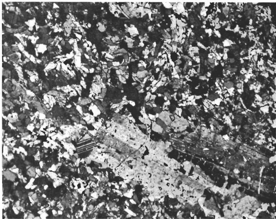
Fig. 68. Andesinporfyr. I en mellanmassa av andesin (huvudsakligen vita korn) och amfibol (huvudsakligen gråsvarta eller svarta listformade korn) förekommer strökorn av andesin. 300 m Ö om sydspetsen av Vaarajärvi. Slipprov. Nic. +, \times 40 .
