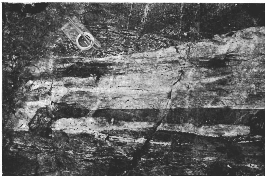
Fig. 21. Granitgång i basisk bandad leptit. Ö om Kaisjärvi. Granite-dike in basic banded leptite. E. of Kaisjärvi.
