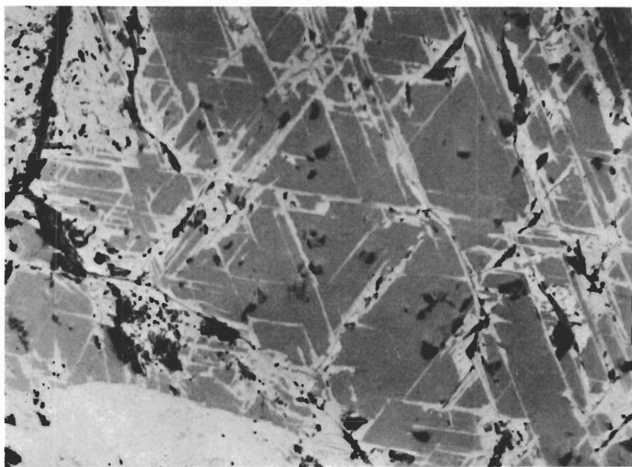
Fig. 42. Svartmalm, något hämatitomvandlad. Hämatit (gråvit) följer oktaederplanen i magnetiten (grå). Svart = apatit? Gruvberget, borrhål 58111, 280.8 m. Polerprov. Vanl. ljus, \times 495 . Magnetite ore, somewhat hematite-altered. Hematite (grey white) follows the octahedral planes in the magnetite (grey). Black = apatite? Gruvberget, drill-hole 58111, 280.8 m. Polished section. Ord. light. \times 495 .
