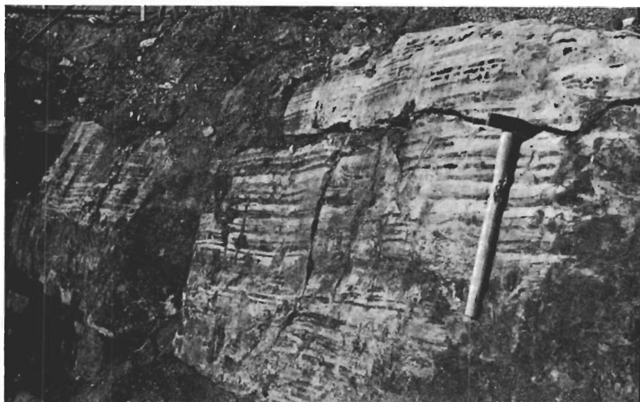
Fig. 6. Skiktning i skapolitfels. 800 m Ö om Hyttjärvi. Bedding in scapolitefels. 800 m E of Hyttjärvi.
