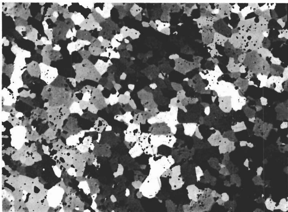
Fig. 47. Tät, massformig blodsten. Hämatit = vit till mörkgrå. Svarta korn mellan hämatiten utgörs av apatit och diopsid. Gruvberget, borrhål 58105, 161.7 m. Polerprov. Nic. +, \times 89 . Dense, non-schistose hematite ore. Hematite = white to dark grey. Dark grains between the hematite are apatite and diopside. Gruvberget, drill-hole 58105, 161.7 m. Polished section. Nic. +, \times 89 .
