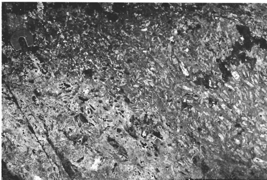
Fig. 26. Andesinporfyrir delvis omvandlad i leukodiabas (i bildens nedre, vänstra hörn). SV om Särkijärvi. Andesine porphyrite partly altered to leucodiabase (in the lower, left part of the picture). SW of Särkijärvi.
