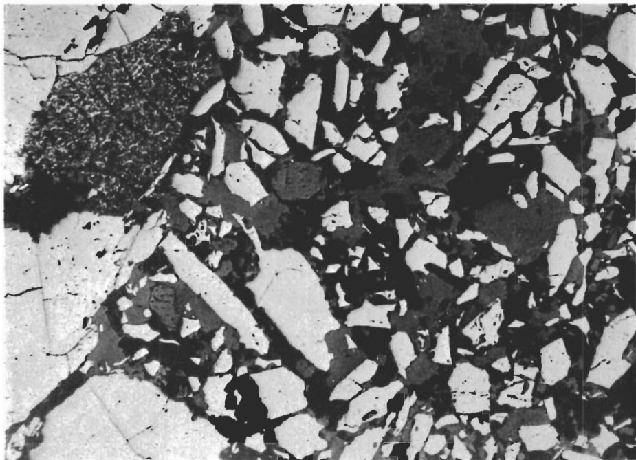
Fig. 54. Fragmentförande blodsten. Fragment av hämatit (vit) i en matrix av klorit (svart) och kvarts (mörkgrå). I övre vänstra hörnet ett martitfragment. Gruvberget, borrhål 23, 44.5 m. Polerprov. Vanl. ljus, \times 47 .
