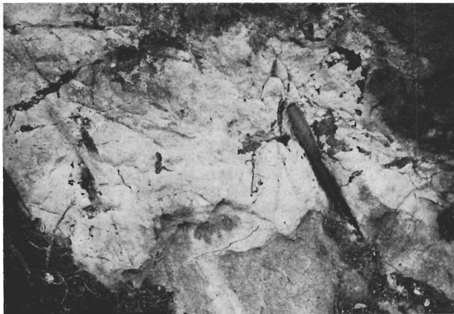
Fig. 25. Leukodiabas med sliror av klorit, amfibol och magnetit liggande i blekt andesinporfyr (underst på bilden). S om Kaisvaara.
