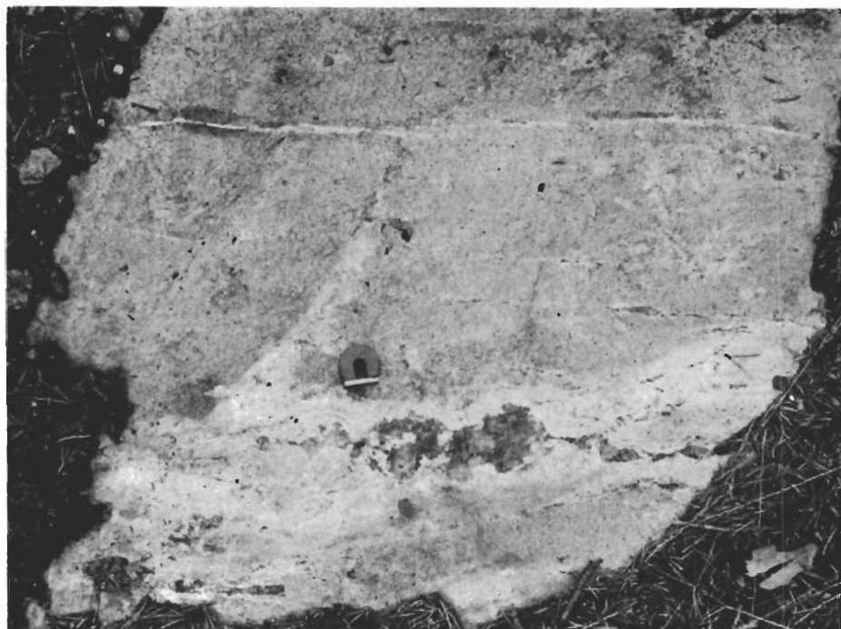
Fig. 17. Andesinporfyrir, delvis blekt, med sliror av amfibol. Ö om Kaisjärvi. Andesine porphyrite, partly bleached, with schlieren of amphibole. E of Kaisjärvi.
