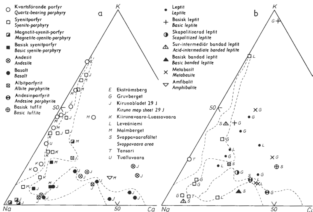
Fig. 2. CaNaK-diagram för vulkaniter (och basiska gångbergarter) i Norrbottens län (a) och Svappavaaraafältet (b).
