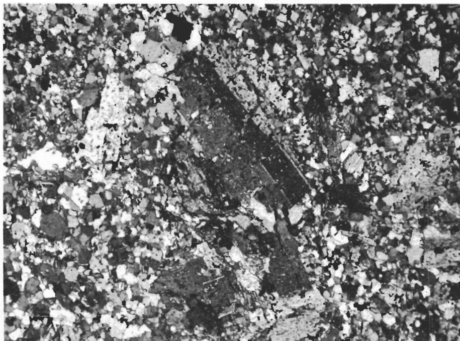
Fig. 60. Syenitporfyr. Albit jämte något biotit och tremolit-aktinolit i mellanmassan. Strökornet består av albit. Gruvberget, borrhål 58117, 55.0 m. Slipprov. Nic. \perp , \times 42 . Syenite-porphyry. Albite with some biotite and tremolite-actinolite make up the matrix. The phenocryst consists of albite. Gruvberget, drill-hole 58117, 55.0 m. Thin section. Nic. \perp , \times 42 .
