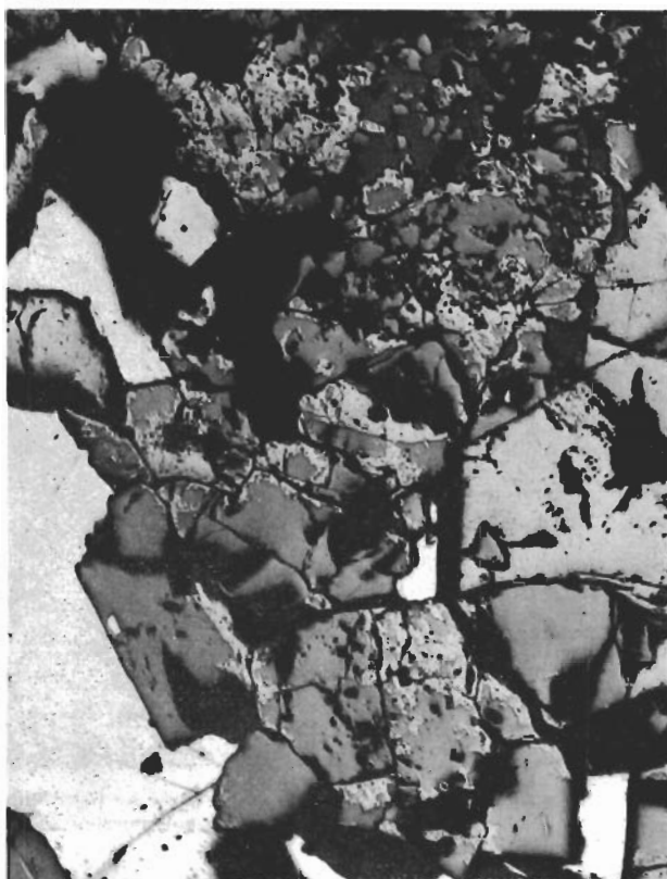
Fig. 58. Malmbreccia. Magnetit (mörkgrå) med hämatit (ljusgrå sliror). Vita eller gråvita, stora korn utgörs av kopparkis. Svarta, oregelbundna fält består av klorit. Gruvberget, borrhål 58114, 220.4 m. Pöllerprov. Vanl. ljus. \times 133 .
