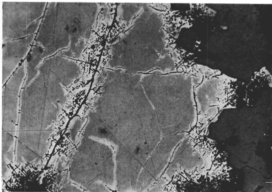
Fig. 31. Kopparmineralisering. Bornit (ljusgrå) omvandlad till kopparglans (vit). Svart - malakit. Till höger klorit (grå) och mikroklin (mörkgrå). Gruvberget, borrhål 15. Polerprov. Nic. +, \times 46 .
