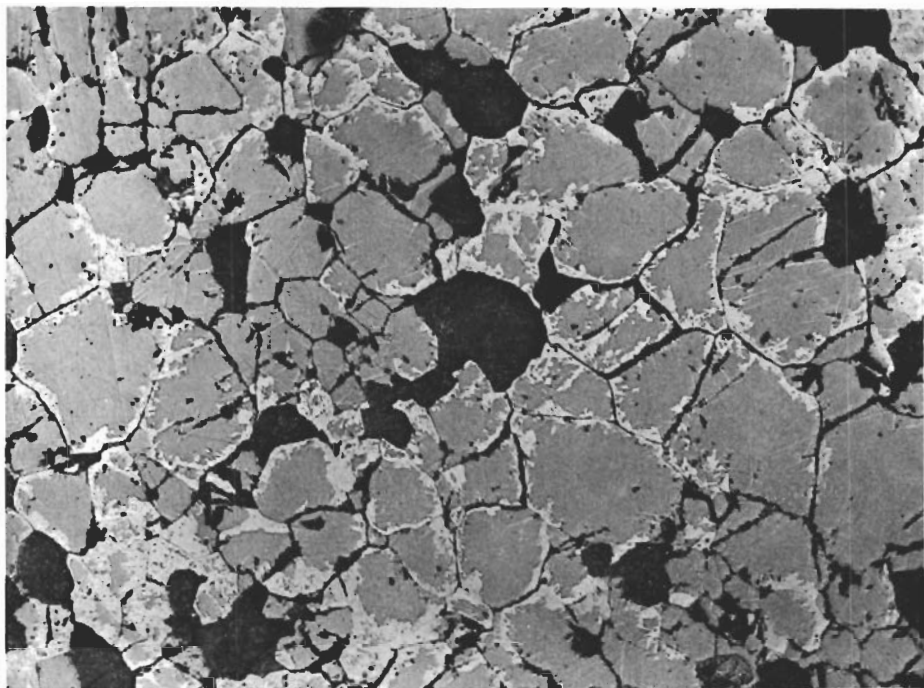
Fig. 41. Svartmalm, något hämatitomvandlad. Hämatit (gråvit) uppträder huvudsakligen kanterna av magnetiten (grå), i ringa mängd i oktaederplanen. Svart = diopsid och limonit. NÖ om Storgruverymningen. Polerprov. Vanl. ljus, \times 142 .
