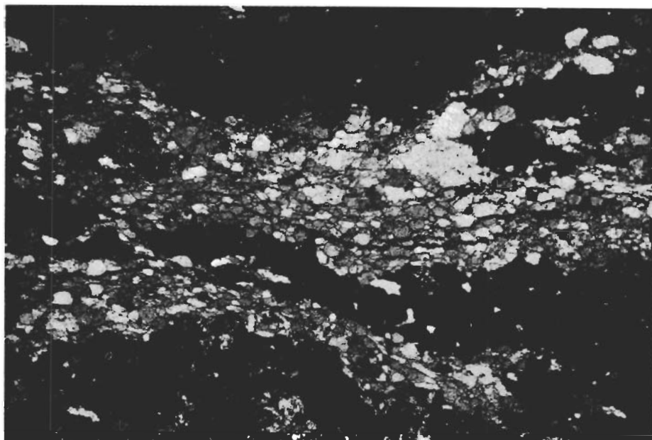
Fig. 44. Apatitslirig svartmalm. Magnetit = svart. Apatit = vit och ljusgrå. I övre, vänstra hörnet ett epidotkorn (gråsvart). NÖ om Storgruverymningen. Slippöv. Nic. +, × 40. Magnetite ore with veins of apatite. Magnetite = black. Apatite = white and light grey. In the upper, left corner a grain of epidote (greyish black). NE of Storgruverymningen. Thin section. Nic. +, × 40.
