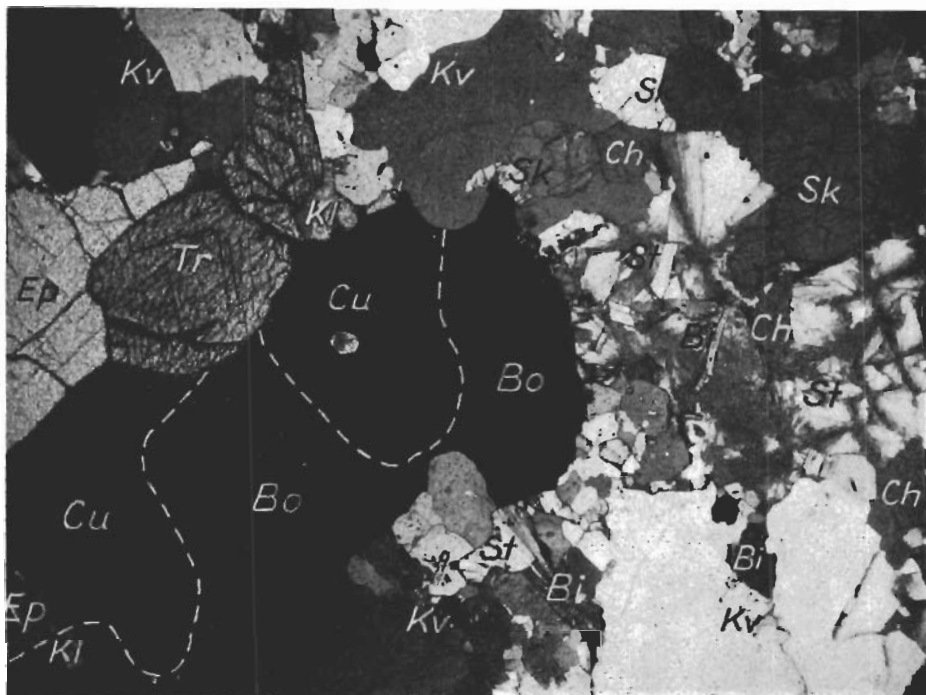
Fig. 28. Kopparmineralisering. Bornit (Bo) och kopparkis (Cu) omgivna av epidot (Ep), kvarts (Kv), skapolit (Sk), stilbit (St) och tremolit-aktinolit (Tr) jämte små mängder biotit (Bi), chabazit (Ch) och klorit (Kl). Gruvberget, borrhål 58102, 19.9 m. Slippöv. Nic. +, \times 32 . Copper mineralization. Bornite (Bo) and chalcopyrite (Cu) are surrounded by epidote (Ep), quartz (Kv), scapolite (Sk), stilbite (St) and tremolite-actinolite (Tr) with small amounts of biotite (Bi), chabazite (Ch) and chlorite (Kl). Gruvberget, drill-hole 58102, 19.9 m. Thin section. Nic. +, \times 32 .
