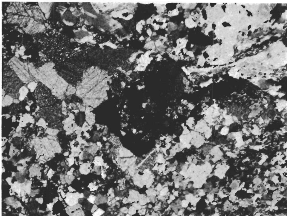
Fig. 27. Kopparmineralisering. I en leptit ligger en slira av kopparkis med något bornit (svarta korn i mitten av bilden), kalcit (grå till gråvita korn till vänster om sulfiderna) och skapolit (i övre, högra hörnet). Runt sulfiderna finns epidot och tremolit-aktinolit (mörkgrå korn).
