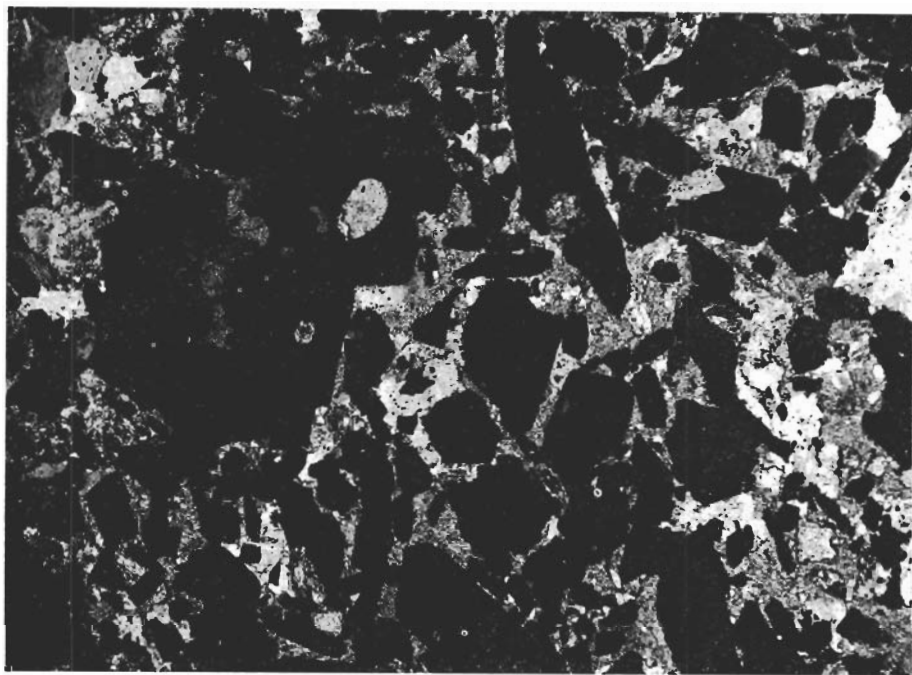
Fig. 53. Fragmentförande blodsten. Fragment av hämatit (svart) i en matrix av klorit (grå) och kvarts (vit). I det stora fragmentet till vänster två runda korn av apatit (ljusgrå). Gruvberget, borrhål 58101, 117.9 m. Slipprov. Nic. +, \times 40 .
