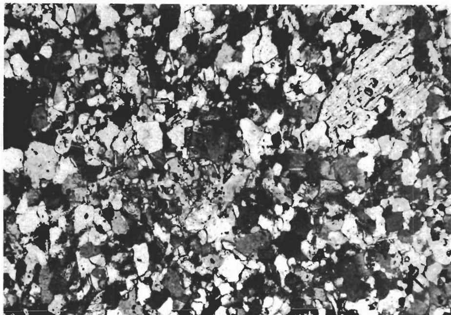
Fig. 56. Leptit, Andesin och kvarts (båda vita till ljusgrå) jämte något biotit (grå). I övre högra hörnet ett korn av tremolit-aktinolit. Små svarta korn består av magnetit. Gruvberget, borrhål 58115, 44.5 m. Slipprov. Nic. +, \times 60 .
