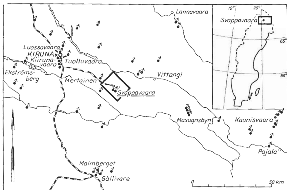
Fig. 1. Karta som visar läget av Svappavaarafältet. Map showing location of the Svappavaara area.
