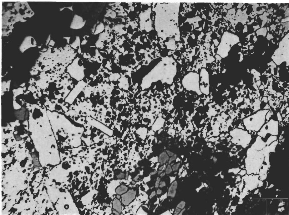
Fig. 43. Hämatitförande svartmalm. I magnetit (gråvit) ligger listformade korn av hämatit (gråvit och med relief). Mindre listformade korn utgörs av apatit (grå). De svarta fläckarna består av epidot och amfibol. Gruvberget, borrhål 18, 14.8 m. Polerprov. Vanl. ljus, \times 72 . Hematite-bearing magnetite ore. In the magnetite (grey white) lie lath-like grains of hematite (grey white and with relief). Smaller lath-like grains consist of apatite (grey). Black patches are epidote and amphibole. Gruvberget, drill-hole 18, 14.8 m. Polished section. Ord. light, \times 72 .
