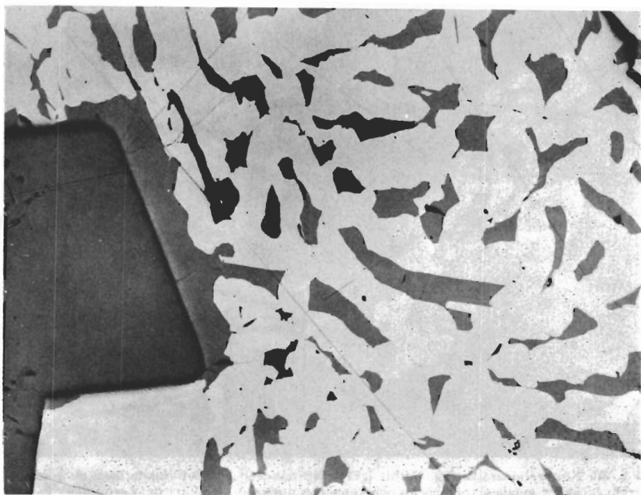
Fig. 29. Kopparmineralisering. Kopparkis (ljusgrå) med lameller av bornit (grå). Till vänster ett korn av magnetit (mörkgrå). Gruvberget, borrhål 15. Polerprov. Vanl. ljus, \times 50 . Copper mineralization. Chalcopyrite (light grey) with lamellae of bornite (grey). To the left a grain of magnetite (dark grey). Gruvberget, drill-hole 15. Polished section. Ord. light, \times 50 .
