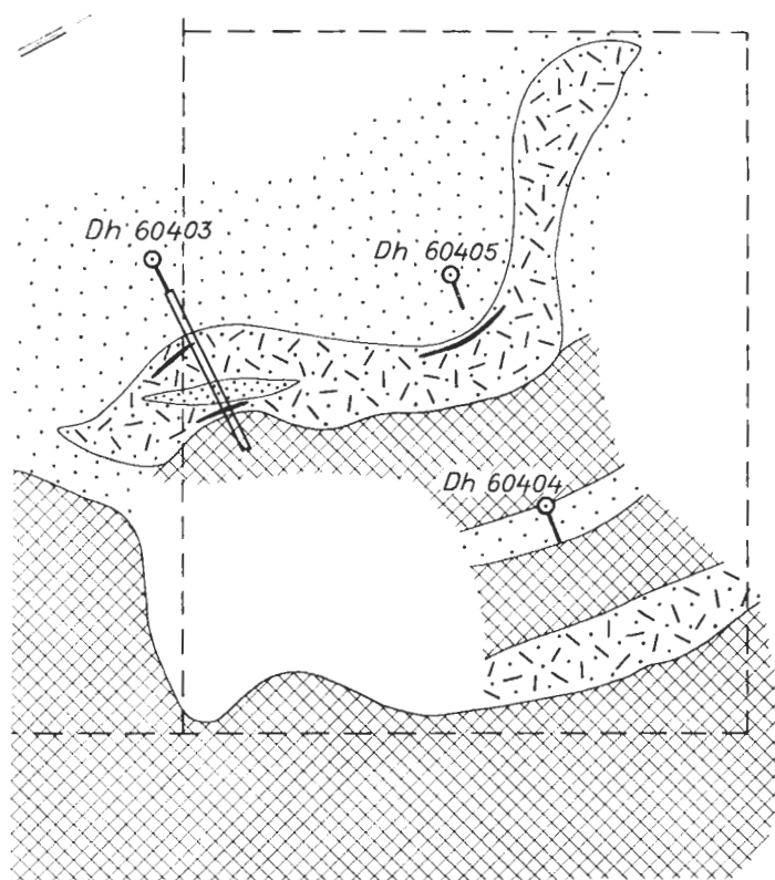
Fig. 77. Karta över Tansari järnmalmsfyndighet. Sketch map of the iron ore deposit at Tansari.
