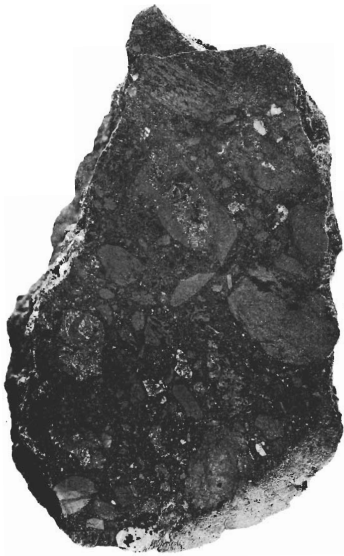
Fig. 52. Fragmentförande blodsten. Gruvberget. Naturlig storlek. Fragment-bearing hematite ore. Gruvberget. Nat. size.
