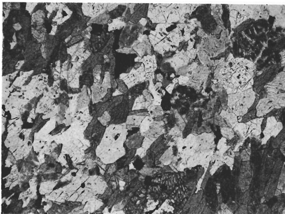
Fig. 67. Metabasit. Skapolit (ljusgrå), biotit (grå fjäll) och enstaka korn av diopsid (grå, kraftig relief, utpräglad spaltning). Små svarta korn utgörs av magnetit. Gruvberget, borrhål 61101, 308.5 m. Slipprov. Vanl. ljus. \times 57 .
