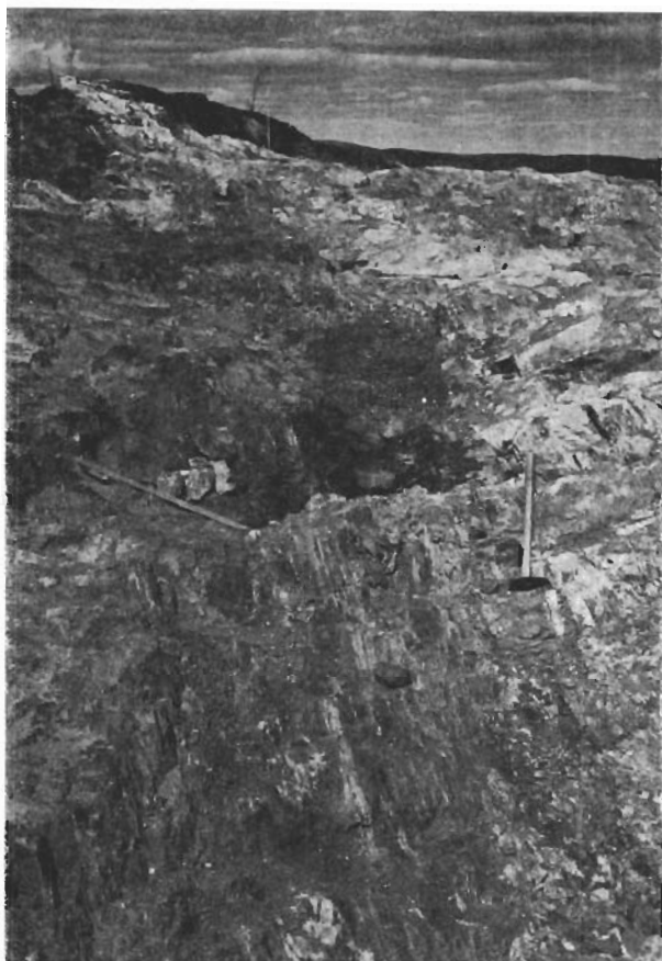
Fig. 34. Krosszon i svartmalm och leptit (till höger om hammaren), NÖ om Storgruverymningen.
