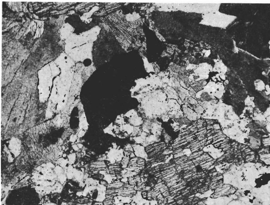
Fig. 72. Skapolitomvandlad leptit. Sekundär slira rik på stilbit (ljusgrå till gråsvarta, radialstråligena aggregat). I mitten av bilden kopparkis (svart); i dess övre, högra del epidot (kraftig relief). I bildens övre och nedre del tremolit-aktinolit (grå, strimmiga korn). Små, ljusgrå korn i stilbiten utgörs av mikroklin. Gruvberget, borrhål 58105, 88.3 m. Slippöv. Nic. +, \times 43 . Scapolitized leptyte. Secondary vein rich in stilbite (light grey to grey, radial arrangement). In the middle of the picture chalcopyrite (black) with epidote to the right. In the upper and lower part of the picture tremolite-actinolite (grey, striped grains). Small, light grey grains in the stilbite are microcline. Gruvberget, drill-hole 58105, 88.3 m. Thin section. Nic. +, \times 43 .
