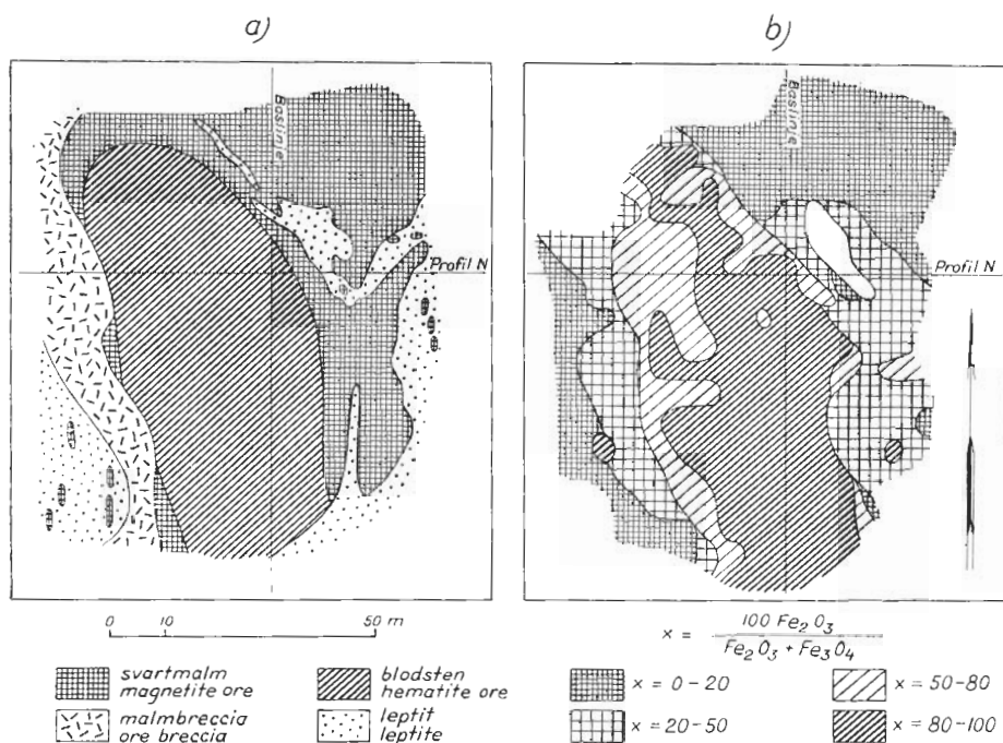
Fig. 50. Karta över övergångszonen mellan svartmalm och blodsten NNÖ om Storgruverymningen: a. geologiska gränser, b. förhållandet hämatit-magnetit på grundval av kemiska analyser.
