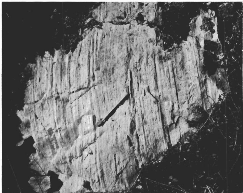
Fig. 12. Sur-intermediär bandad leptit. Ö om Kaisjärvi. Acid-intermediate banded leptite. E of Kaisjärvi.
