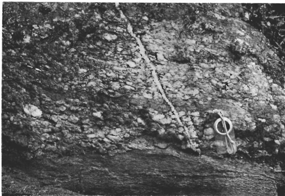
Fig. 8. Konglomerat i kvartsitsandsten. S om Iso Kulujärvi. Conglomerate in quartzitic sandstone. S of Iso Kulujärvi.
