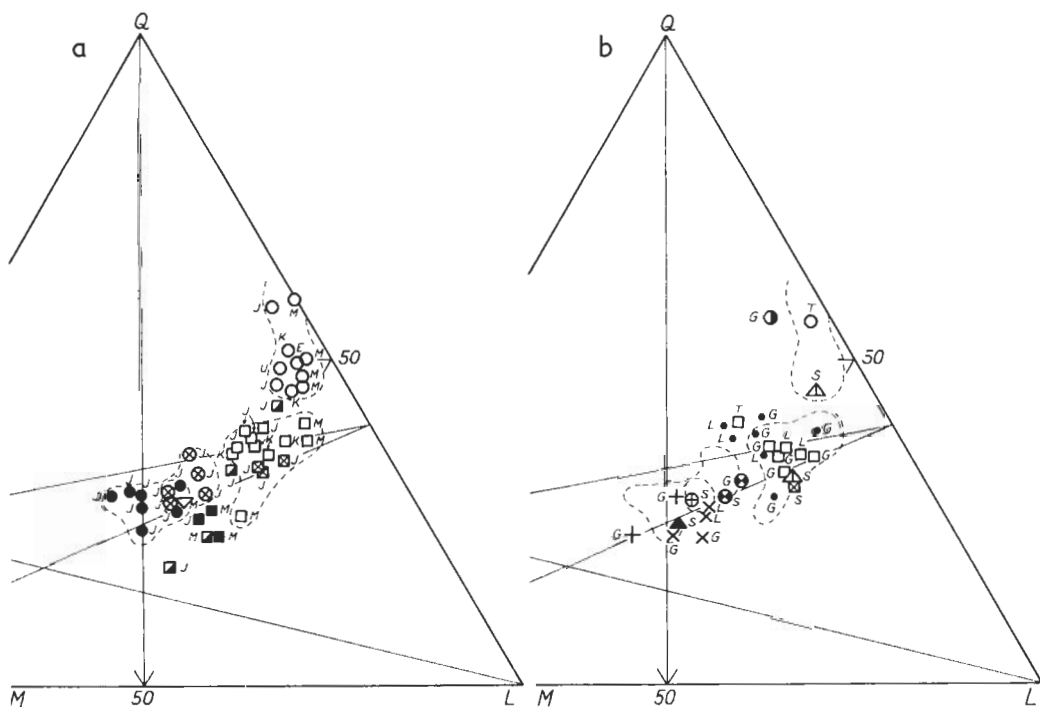
Fig. 3. QLM-diagram för vulkaniter (och basiska gångbergarter) i Norrbottens län (a) och Svappavaarafältet (b). Teckenförklaring se fig. 2.
