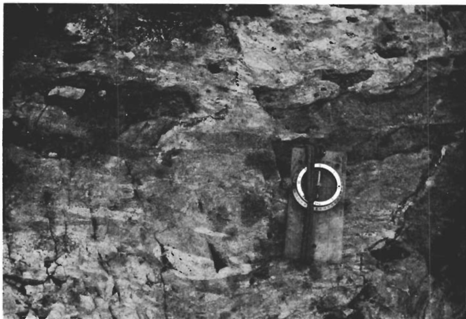
Fig. 13. Konglomerat i sur-intermediär bandad leptit. SÖ om Kaisjärvi. Conglomerate in acid-intermediate banded leptite. SE of Kaisjärvi.
