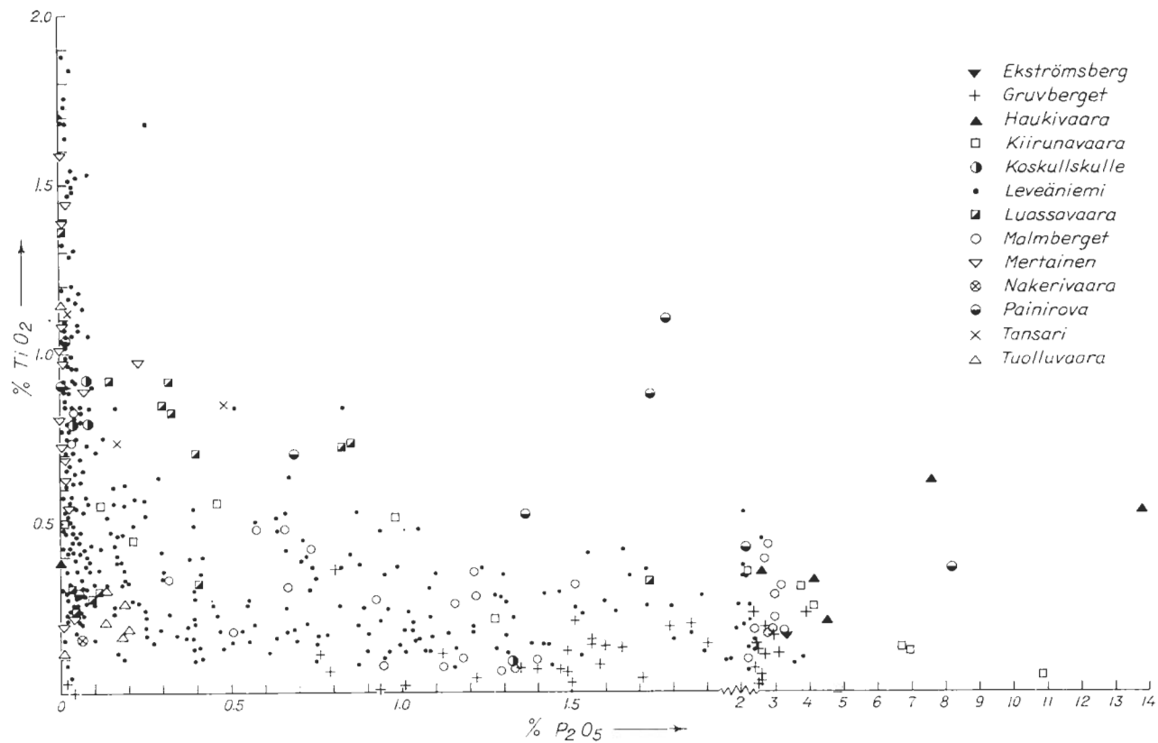
Fig. 83. Halterna av P_2O_5 och TiO_2 i apatitjärnmalm i Norrbotten. Vikt %. P_2O_5 and TiO_2 values in apatite iron ores of Norrbotten. Weight %.
