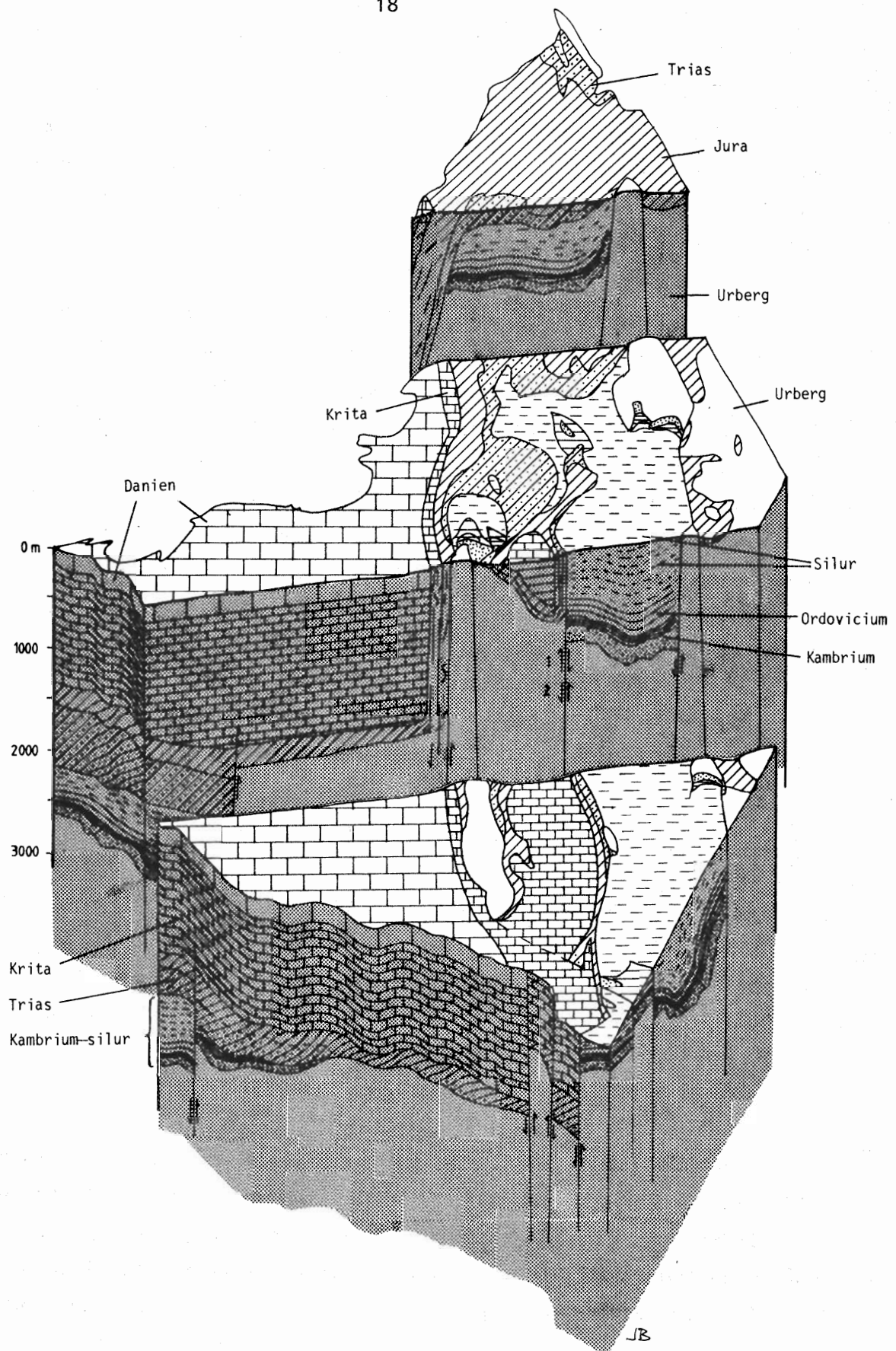
Uppsnittat blockdiagram visande berggrunden i sydvästra Skåne
