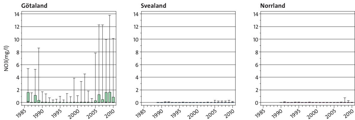
Figur 3. Nitrathalter i markvatten. Alla analyser från IVLs provtagningsnät. Boxplot med 10-, 25-, 50-, 75- och 90-percentiler.
