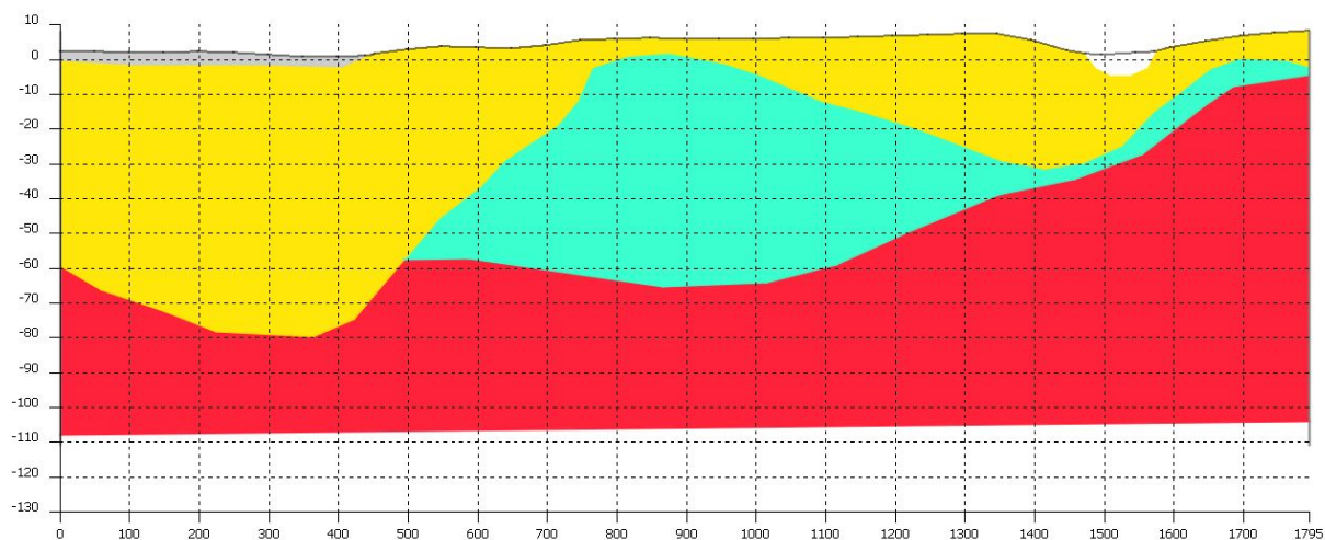
Figur 2. En tvärsektion från väst-öst i mitten av området.
