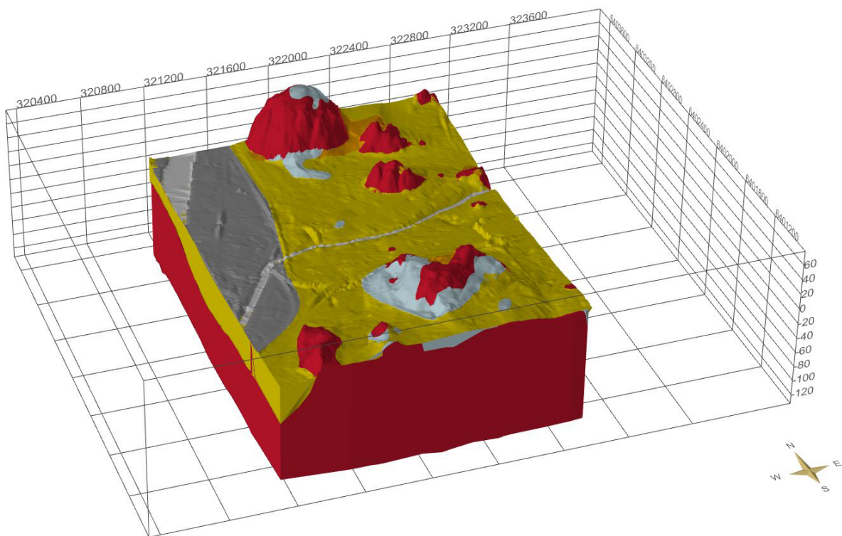
Figur 3. Den färdiga modellen som den visas i 3D-fönstret i programmet Subsurface viewer.
